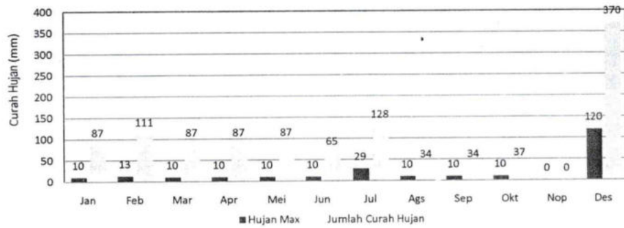
GRAFIK : HUJAN MAX DAN JUMLAH HUJAN BULANAN (MM) 2019 STASIUN : BOU- LINTAU BUO
