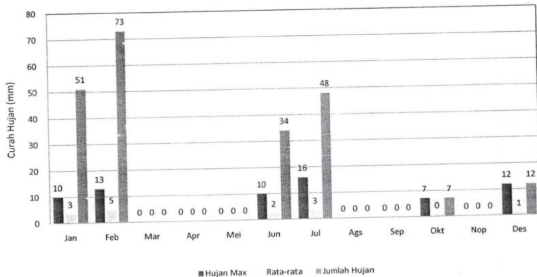
GRAFIK : CURAH HUJAN PRIODE ( 15 HARIAN 1) 2019 STASIUN : BUO- LINTAU BUO
