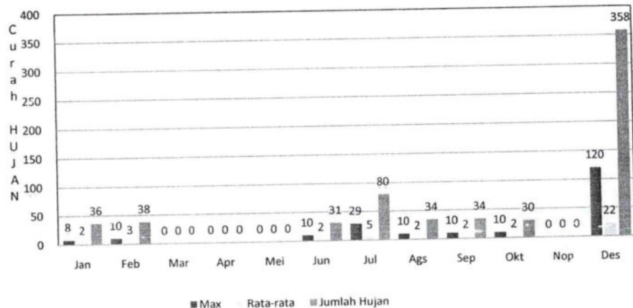
GRAFIK : CURAH HUJAN PRIODE (15 HARIAN 2) 2019 STASIUN : BUO- LINTAU BUO
