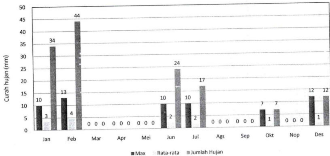
GRAFIK : CURAH HUJAN PRIODE 10 HARIAN 1 (MM) STASIUN : GANGGO MUDIK - BONJOL
