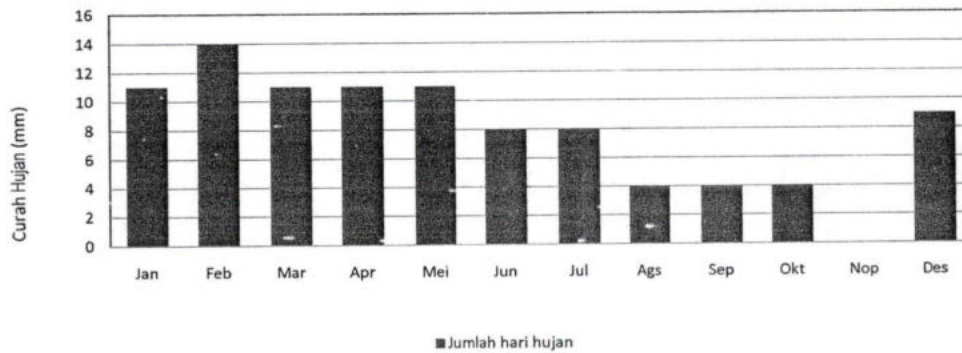
GRAFIK : JUMLAH HARI HUJAN (MM) 2019 STASIUN : BUO - LINTAU BUO
