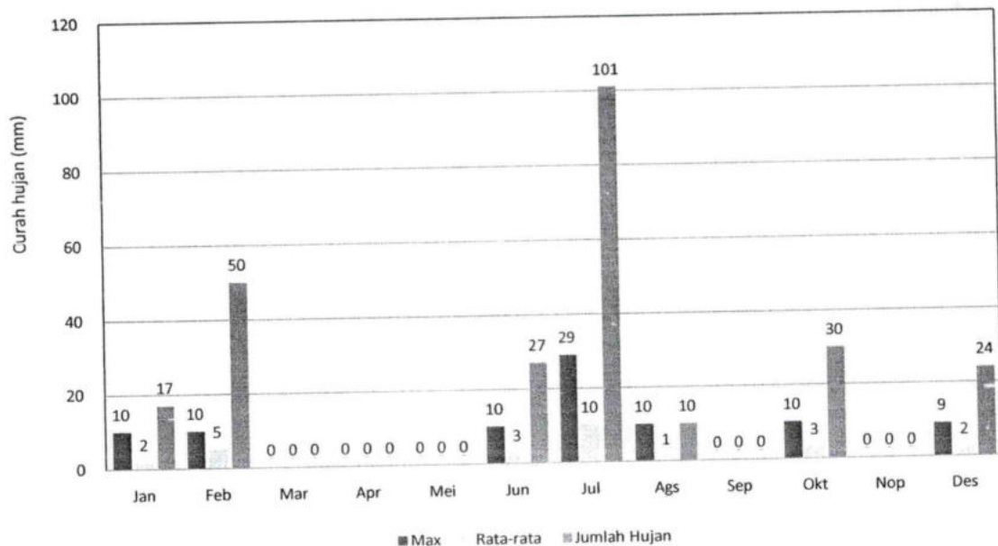
GRAFIK : CURAH HUJAN PRIODE 10 HARIAN 2 (MM) STASIUN : GANGGO MUDIK - BONJOL
