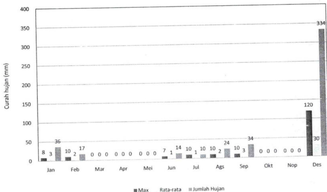
GRAFIK : CURAH HUJAN PRIODE 10 HARIAN 3 (MM) STASIUN : GANGGO MUDIK - BONJOL
