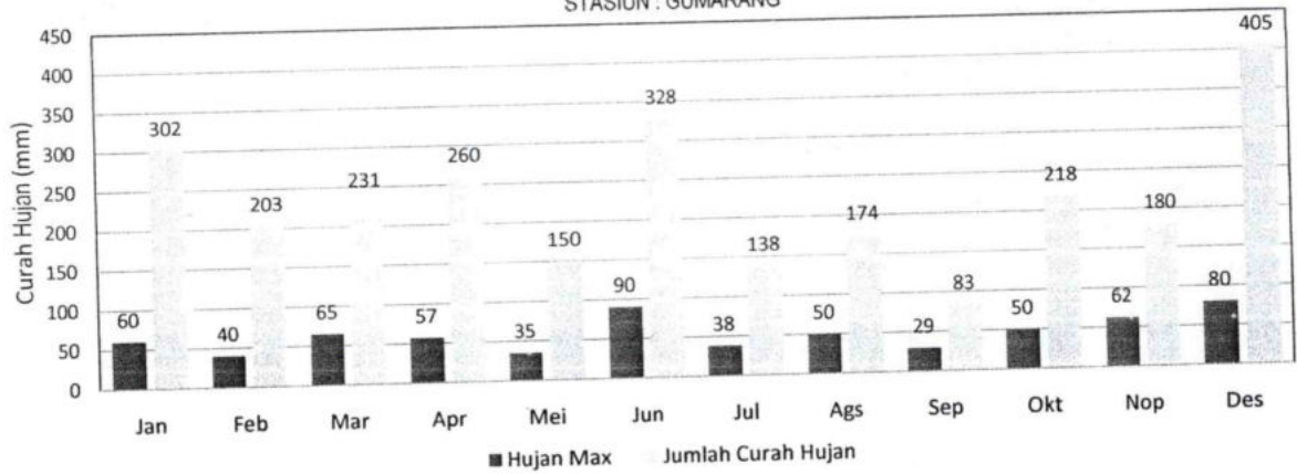
GRAFIK : HUJAN MAX DAN JUMLAH HUJAN BULANAN (MM) 2019
