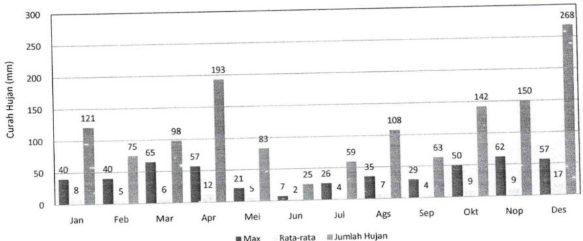
GRAFIK : CURAH HUJAN PRIODE (15 HARIAN 2) 2019 STASIUN : GUMARANG
