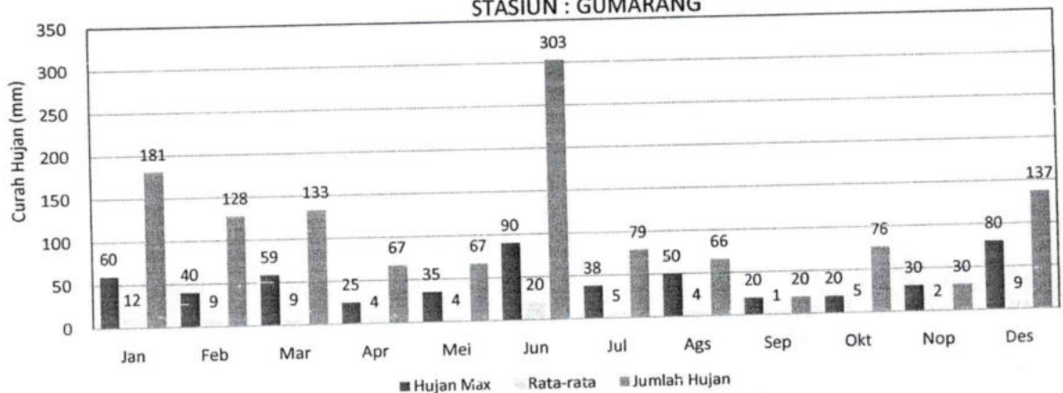
GRAFIK : CURAH HUJAN PRIODE ( 15 HARIAN 1) 2019 STASIUN : GUMARANG
