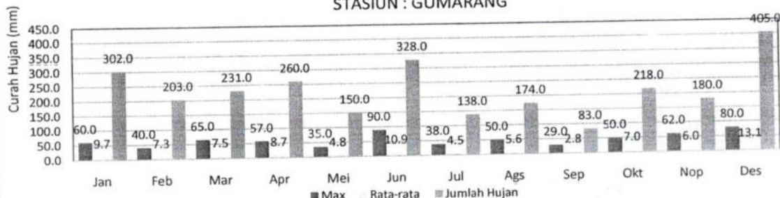
GRAFIK : CURAH HUJAN PRIODE BULANAN (MM) 2019 STASIUN : GUMARANG
