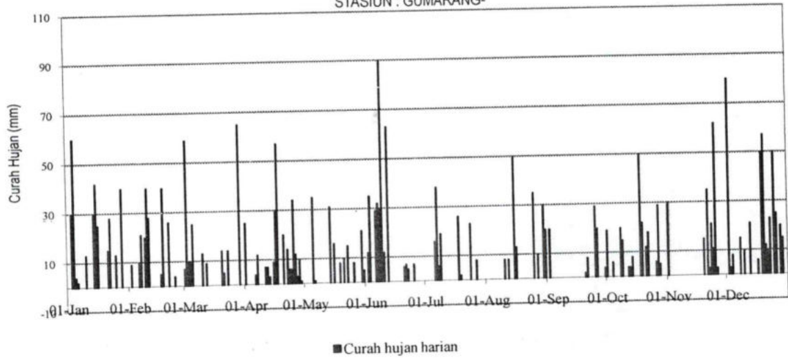
STATISTIK CURAH HUJAN HARIAN (MM) 2019 STASIUN : GUMARANG-
