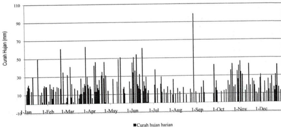
GRAFIK : HUJAN MAX DAN JUMLAH HUJAN BULANAN (MM) 2019 STASIUN : LADANG PADI
