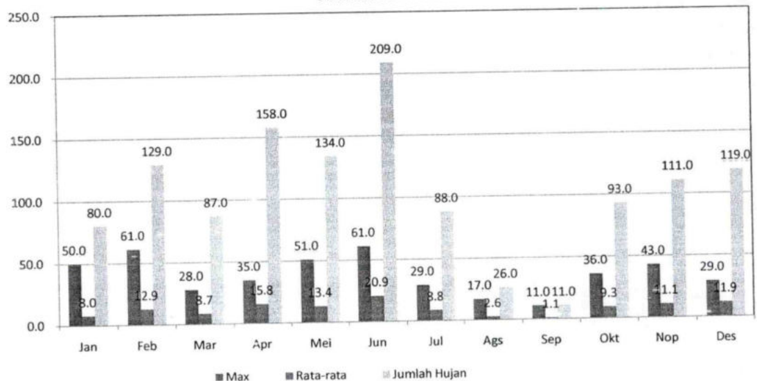
GRAFIK : CURAH HUJAN PRIODE 10 HARIAN 2 (MM) STASIUN : LADANG PADI
