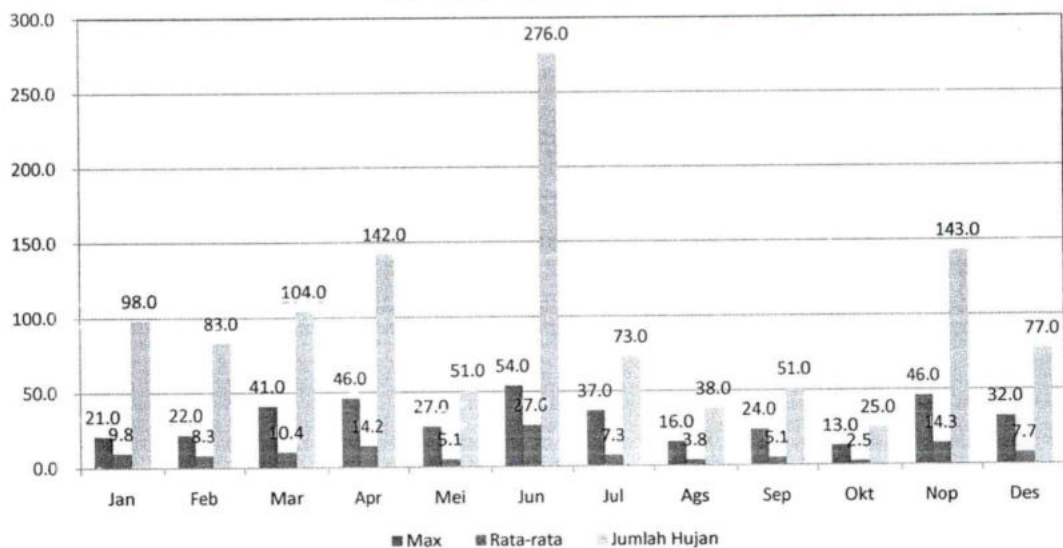
GRAFIK : CURAH HUJAN PRIODE 10 HARIAN 1 (MM) STASIUN : LADANG PADI
