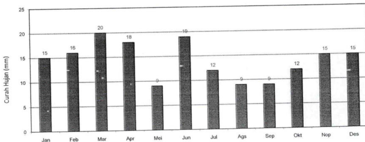
GRAFIK : JUMLAH HARI HUJAN (MM) 2019 STASIUN : LADANG PADI
