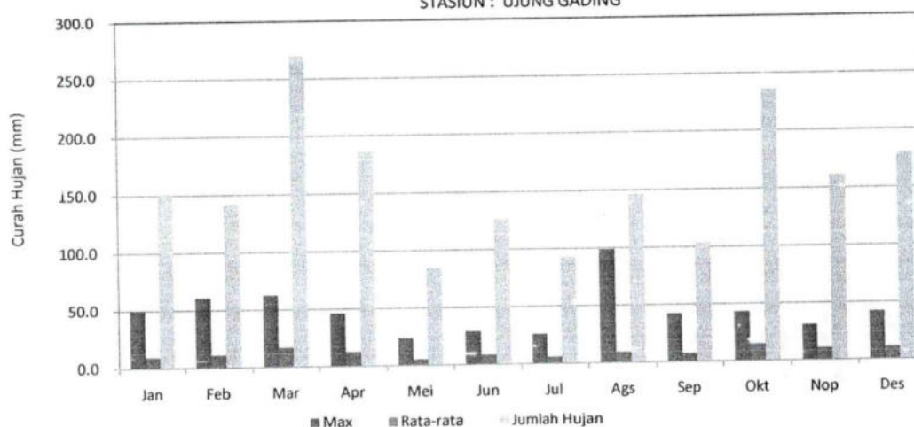
GRAFIK : CURAH HUJAN PRIODE (15 HARIAN 2) 2019 STASIUN : UJUNG GADING
