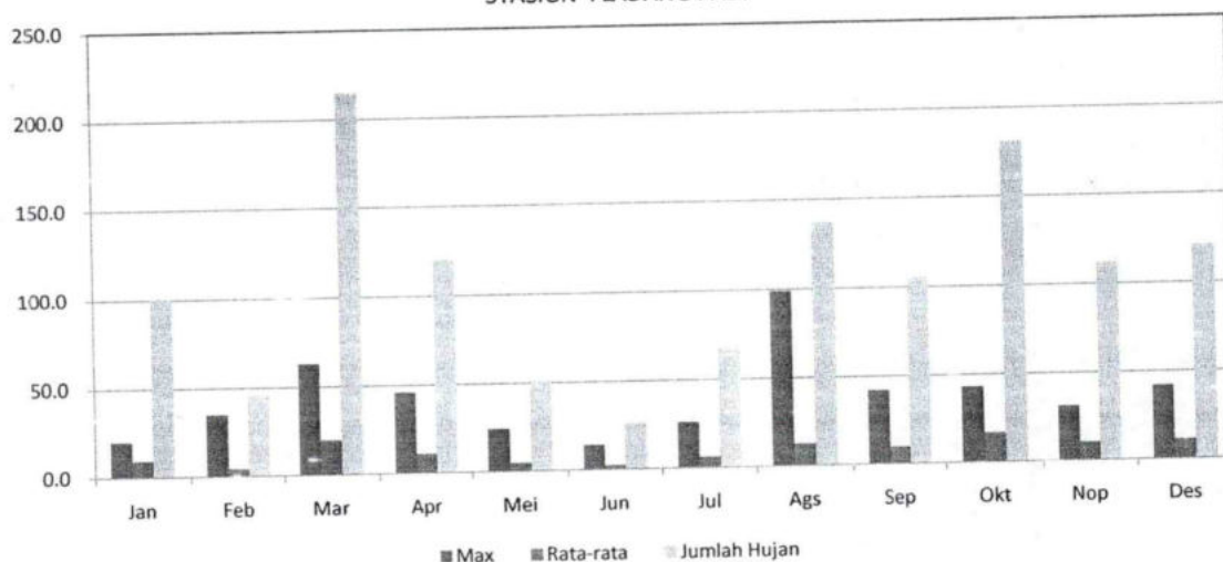
GRAFIK : CURAH HUJAN PRIODE 10 HARIAN 3 (M:M) STASIUN : LADANG PADI
