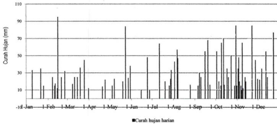
STATISTIK CURAH HUJAN HARIAN (MM) 2018 STASIUN : SANTOK
