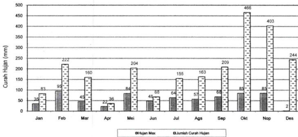
GRAFIK : HUJAN MAX DAN JUMLAH HUJAN BULANAN (MM) 2018 STASIUN : SANTOK
