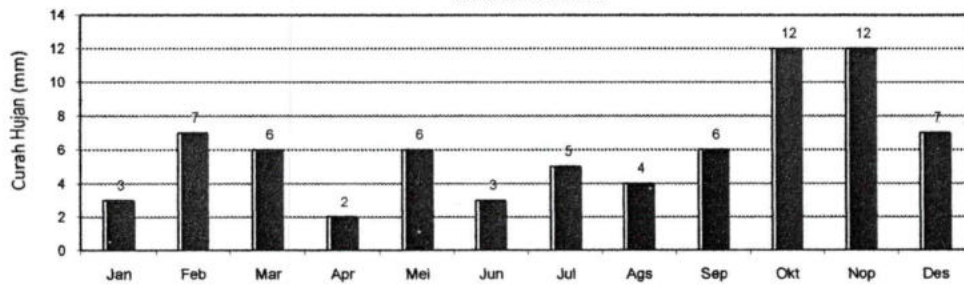
GRAFIK : JUMLAH HARI HUJAN (MM) 2018 STASIUN : SANTOK
