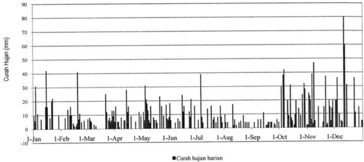
GRAFIK : HUJAN MAX DAN JUMLAH HUJAN BULANAN (MM) 2019 STASIUN : SONTANG
