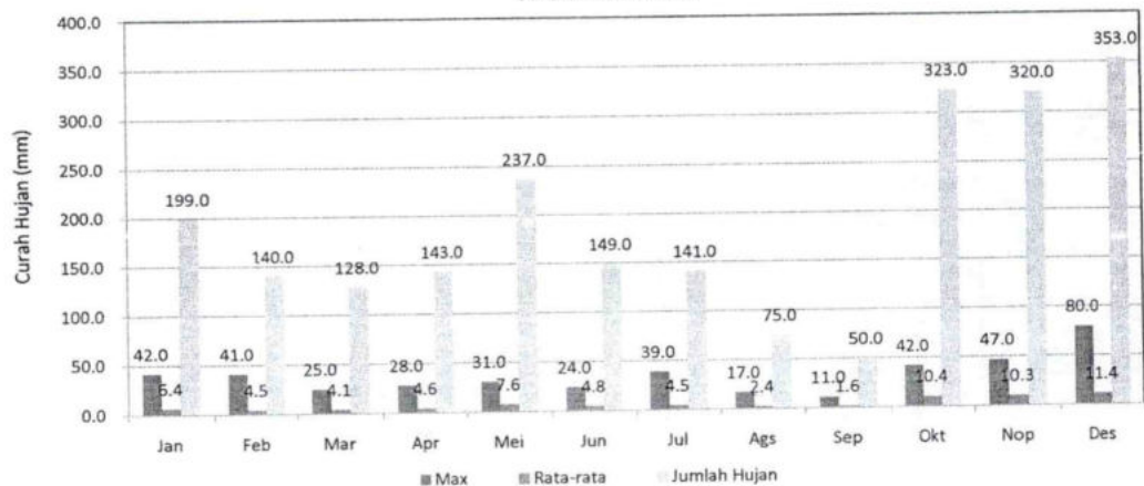
GRAFIK : CURAH HUJAN PRIODE BULANAN (MM) 2019 STASIUN : SONTANG
