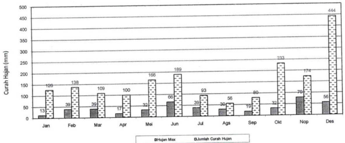
GRAFIK : HUJAN MAX DAN JUMLAH HUJAN BULANAN (MM) 2019 STASIUN : SULIKI
