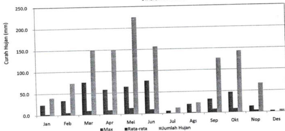
GRAFIK : CURAH HUJAN PRIODE (15 HARIAN 2) 2018 STASIUN : SUMANI
