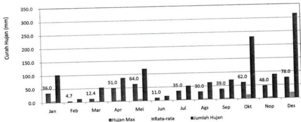
GRAFIK : CURAH HUJAN PRIODE ( 15 HARIAN 1) 2017 STASIUN : SUMANI
