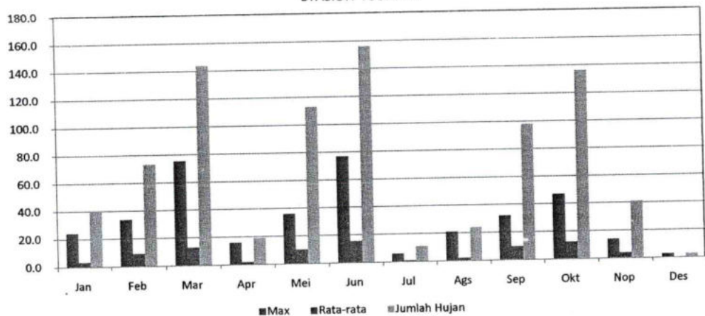
GRAFIK : CURAH HUJAN PRIODE 10 HARIAN 3 (MM) STASIUN : SUMANI
