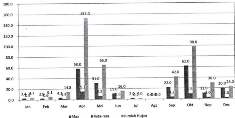
GRAFIK : CURAH HUJAN PRIODE 10 HARIAN 2 (MM) STASIUN : SUMANI
