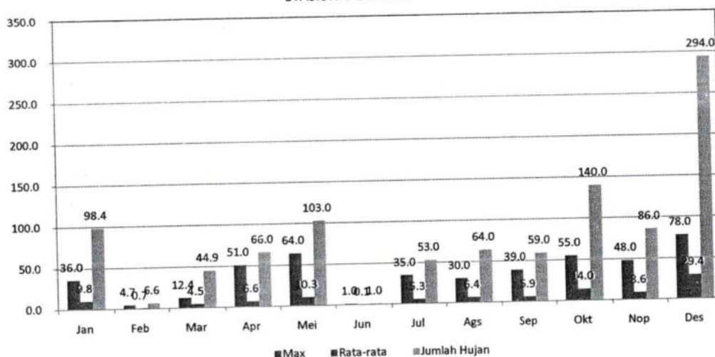
GRAFIK : CURAH HUJAN PRIODE 10 HARIAN 1 (MM) STASIUN : SUMANI
