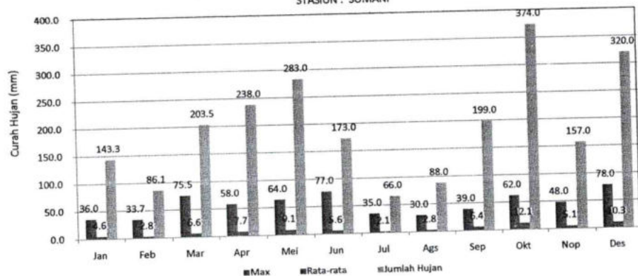
GRAFIK : CURAH HUJAN PRIODE BULANAN (MM) 2018 STASIUN : SUMANI
