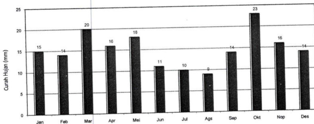
GRAFIK : JUMLAH HARI HUJAN (MM) 2018 STASIUN : SUMANI
