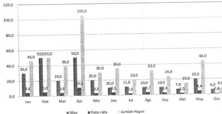
GRAFIK : CURAH HUJAN PRIODE 10 HARIAN 2 (MM) STASIUN : CANDUANG
