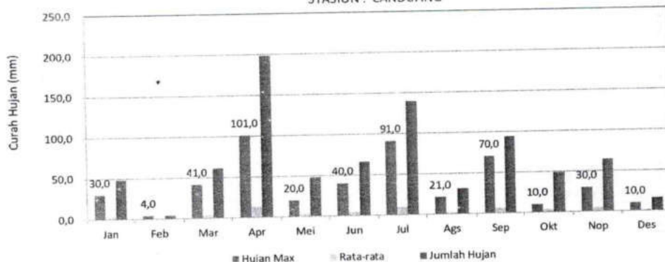
GRAFIK : CURAH HUJAN PRIODE ( 15 HARIAN 1) 2020 STASIUN : CANDUANG
