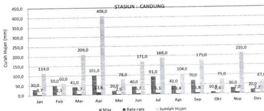
GRAFIK : CURAH HUJAN PRIODE BULANAN (MM) 2020
