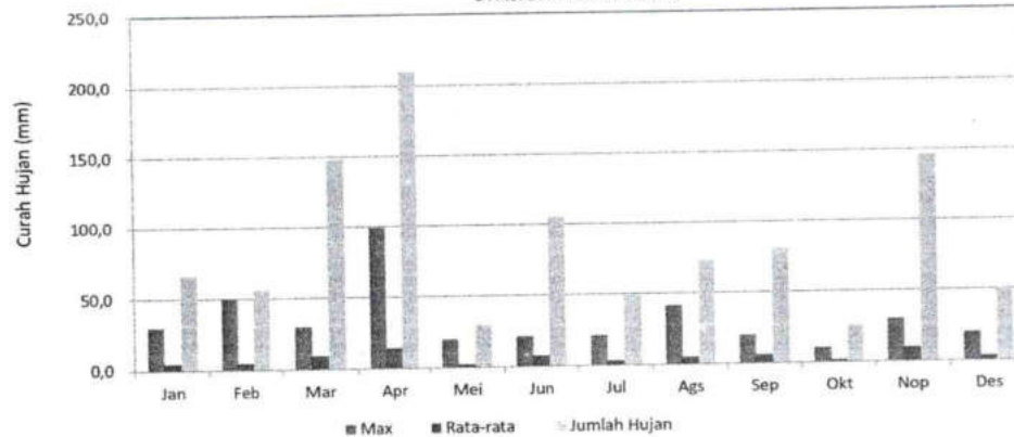
GRAFIK : CURAH HUJAN PRIODE (15 HARIAN 2) 2020 STASIUN : CANDUANG
