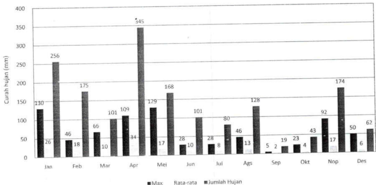
GRAFIK : CURAH HUJAN PRIODE 10 HARIAN 2 (MM) STASIUN : KANDANG IV
