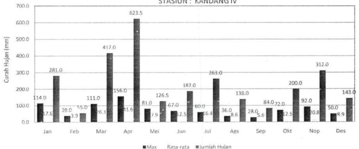
GRAFIK : CURAH HUJAN PRIODE (15 HARIAN 2) 2020
