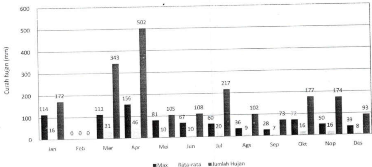
GRAFIK : CURAH HUJAN PRIODE 10 HARIAN 3 (MM) STASIUN : KANDANG IV
