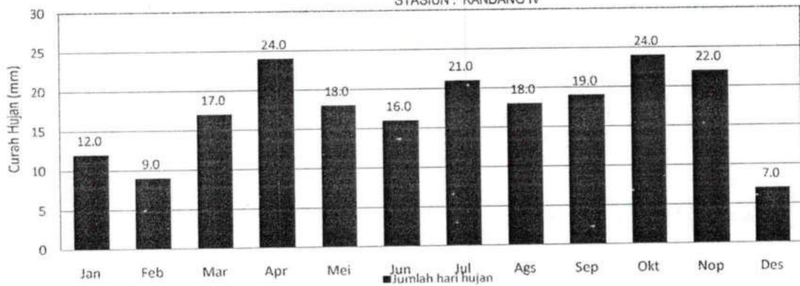
GRAFIK : JUMLAH HARI HUJAN (MM) 2020 STASIUN : KANDANG IV
