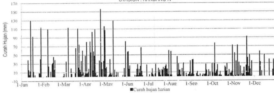
STATISTIK CURAH HUJAN HARIAN (MM) 2020 STASIUN : KANDANG IV
