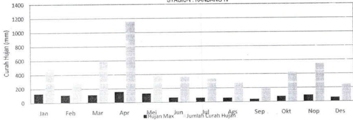
GRAFIK : HUJAN MAX DAN JUMLAH HUJAN BULANAN (MM) 2020 STASIUN : KANDANG IV
