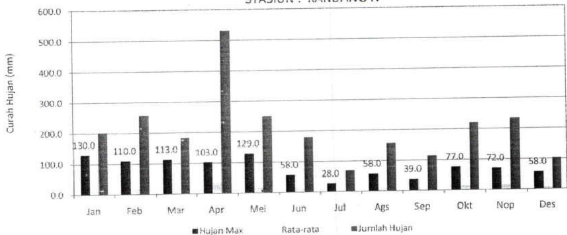
GRAFIK : CURAH HUJAN PRIODE ( 15 HARIAN 1 ) 2020 STASIUN : KANDANG IV
