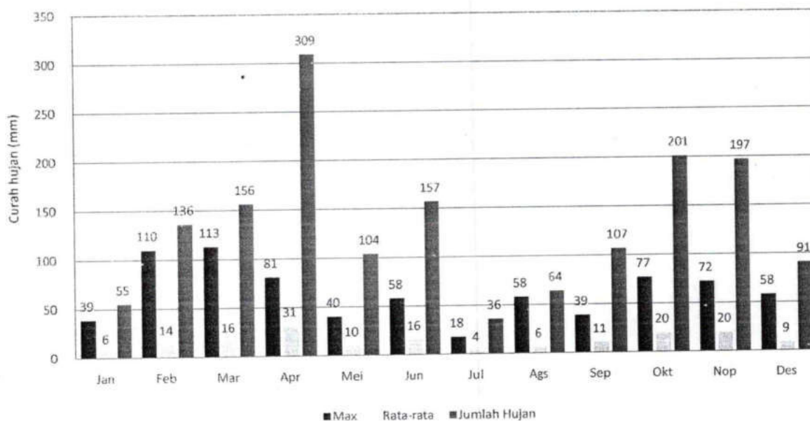
GRAFIK : CURAH HUJAN PRIODE 10 HARIAN 1 (MM) STASIUN : KANDANG IV
