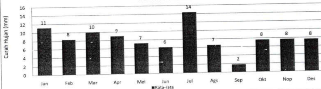
GRAFIK : CURAH HUJAN RATA-RATA BULANAN (MM) 2020 STASIUN : KASANG
