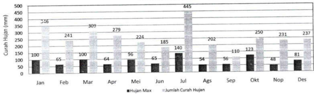
GRAFIK : HUJAN MAX DAN JUMLAH HUJAN BULANAN (MM) 2020 STASIUN : KASANG
