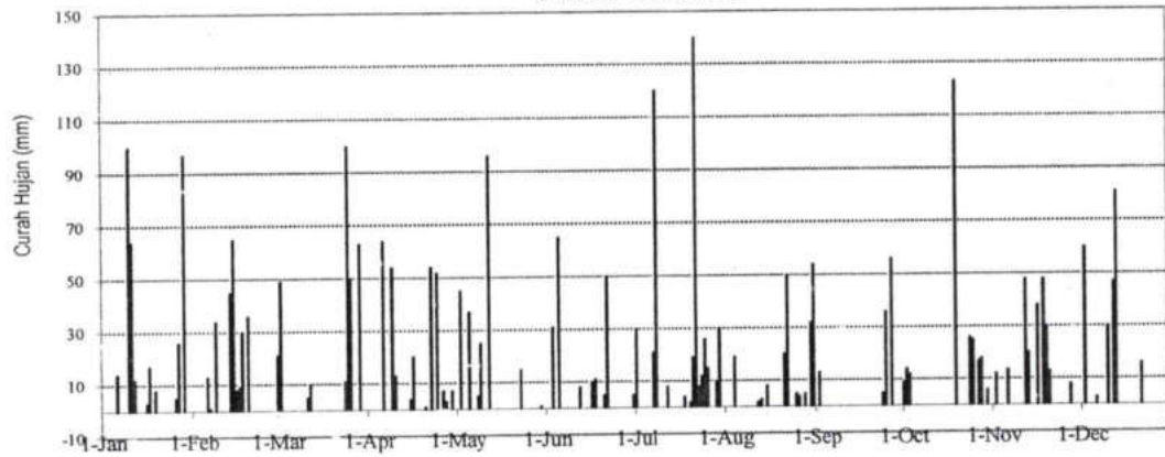
STATISTIK CURAH HUJAN HARIAN (MM) 2020 STASIUN : KASANG
