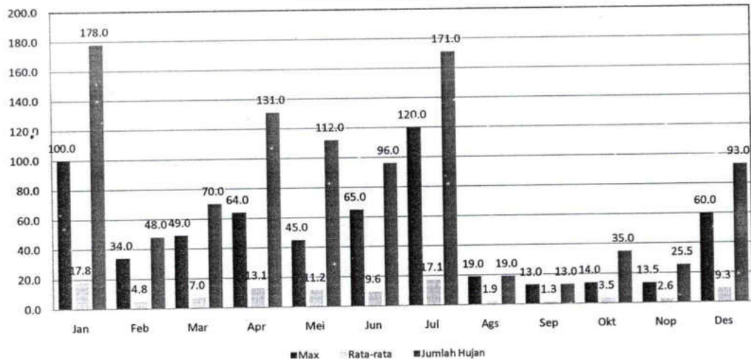
GRAFIK : CURAH HUJAN PRIODE 10 HARIAN 1 (MM) STASIUN : KASANG
