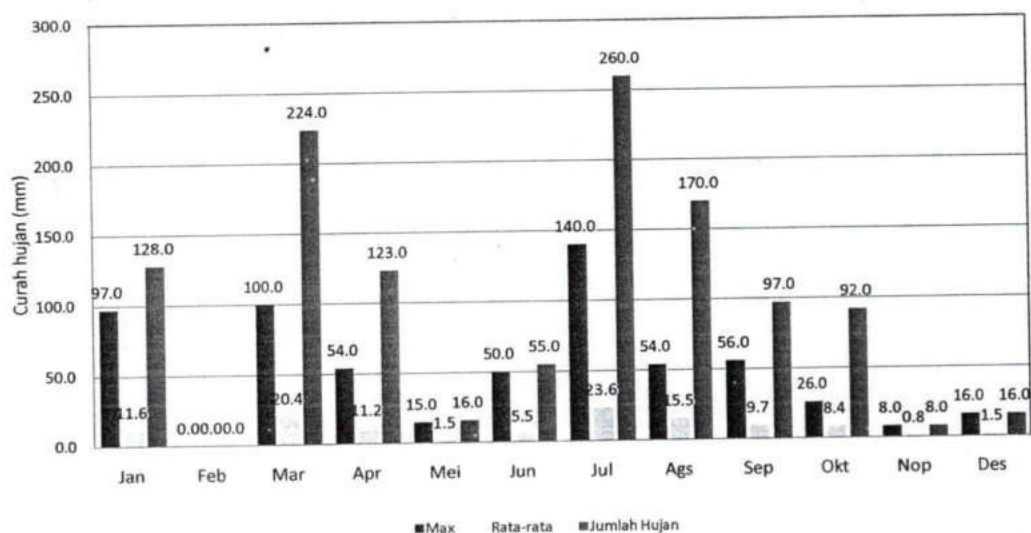
GRAFIK : CURAH HUJAN PRIODE 10 HARIAN 3 (MM) STASIUN : KASANG
