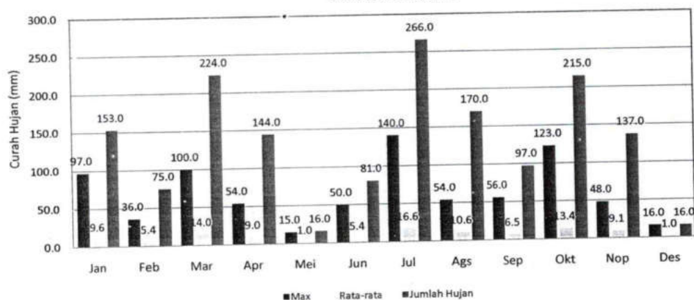
GRAFIK : CURAH HUJAN PRIODE (15 HARIAN 2) 2020 STASIUN : KASANG
