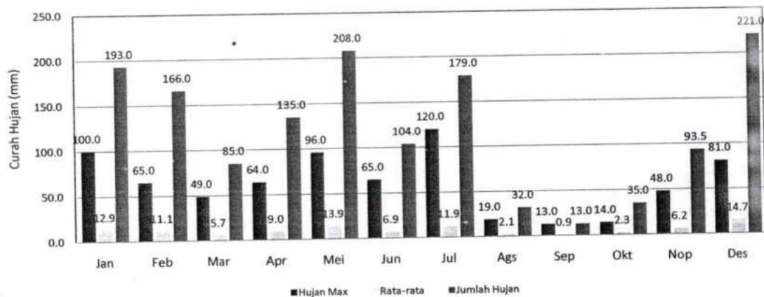
GRAFIK : CURAH HUJAN PRIODE ( 15 HARIAN 1) 2020 STASIUN : KASANG
