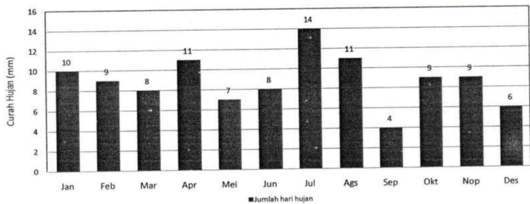
GRAFIK : JUMLAH HARI HUJAN (MM) 2020 STASIUN : KASANG
