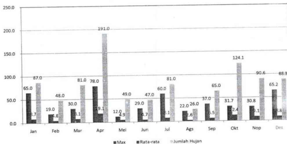
GRAFIK : CURAH HUJAN PRIODE 10 HARIAN 1 (MM) STASIUN : MUARA TANTANG
