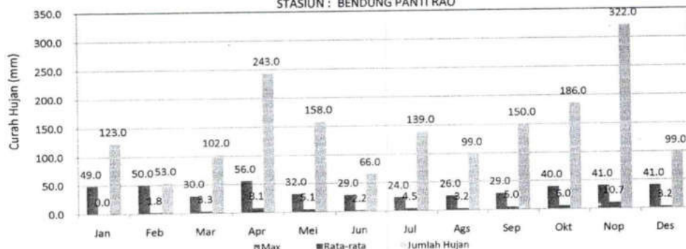
GRAFIK : CURAH HUJAN PRIODE BULANAN (MM) 2020 STASIUN : BENDUNG PANTI RAO
