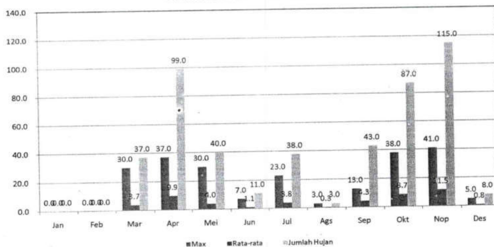
GRAFIK : CURAH HUJAN PRIODE 10 HARIAN 1 (MM) STASIUN : BENDUNG PANTI RAO
