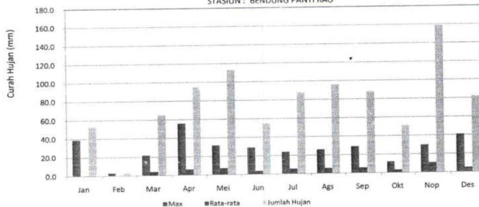
GRAFIK : CURAH HUJAN PRIODE (15 HARIAN 2) 2020 STASIUN : BENDUNG PANTI RAO
