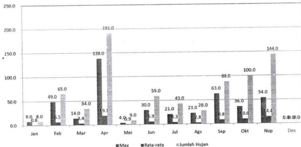
GRAFIK : CURAH HUJAN PRIODE 10 HARIAN 1 (MM) STASIUN : RAO
