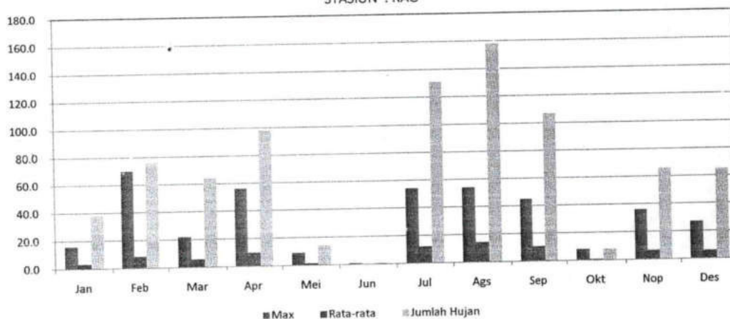
GRAFIK : CURAH HUJAN PRIODE 10 HARIAN 3 (MM) STASIUN : RAO
