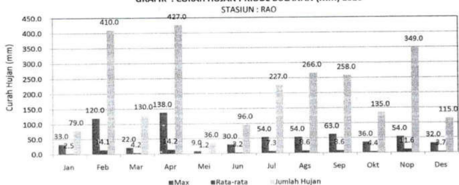
GRAFIK : CURAH HUJAN PRIODE BULANAN (MM) 2020
