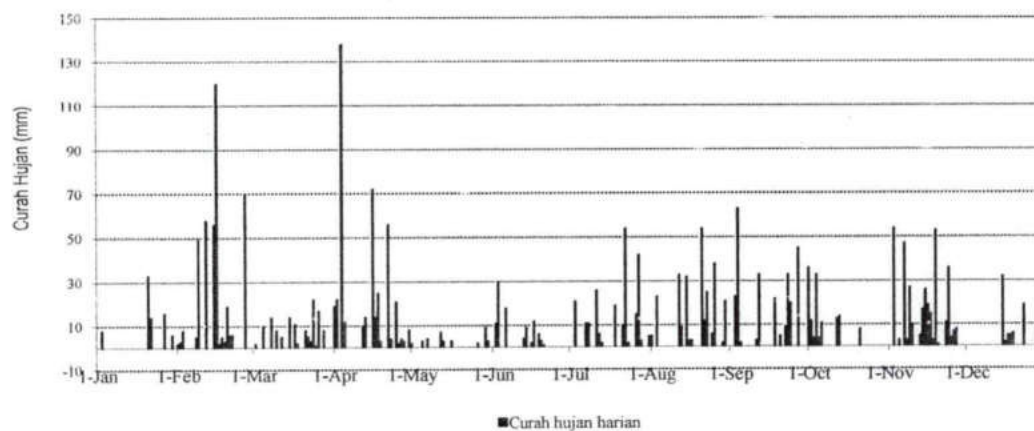
STATISTIK CURAH HUJAN HARIAN (MM) 2020 STASIUN : RAO
