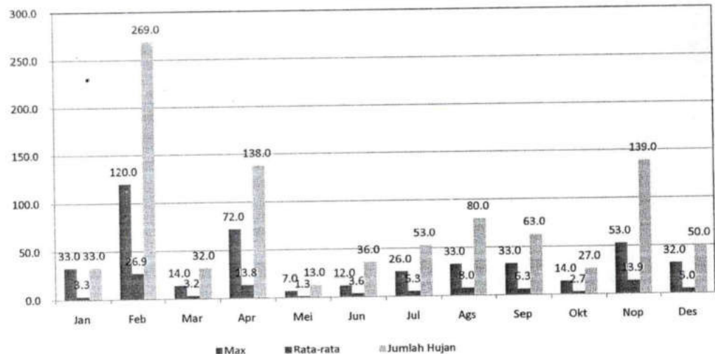
GRAFIK : CURAH HUJAN PRIODE 10 HARIAN 2 (MM) STASIUN : RAO
