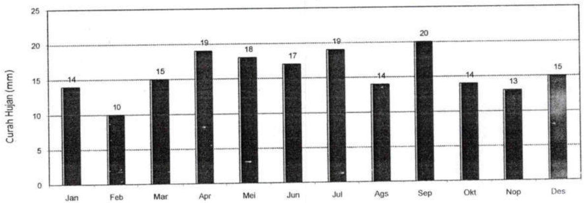
GRAFIK : JUMLAH HARI HUJAN (MM) 2020
