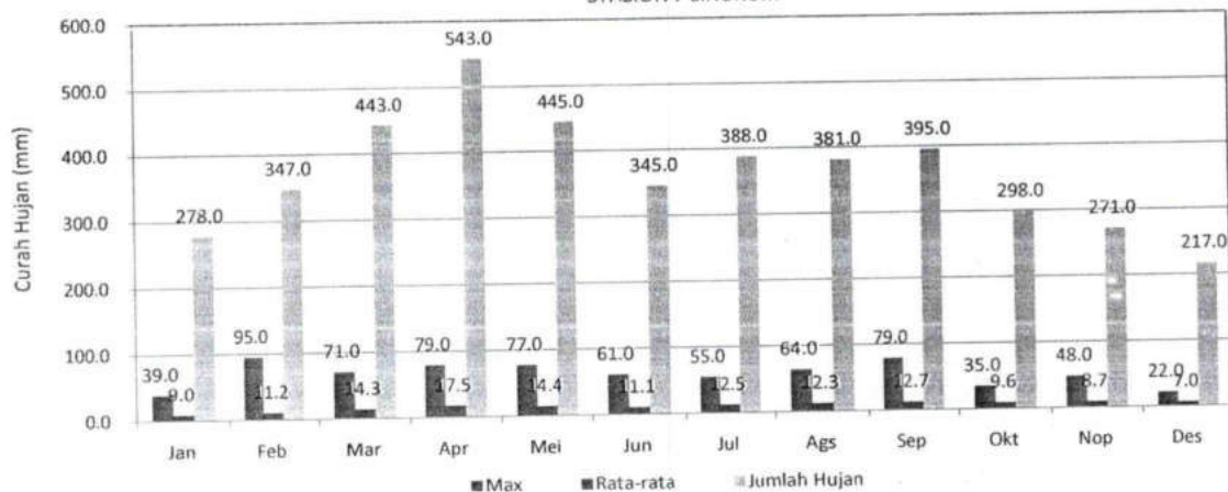
GRAFIK : CURAH HUJAN PRIODE BULANAN (MM) 2020 STASIUN : SINURUIK
