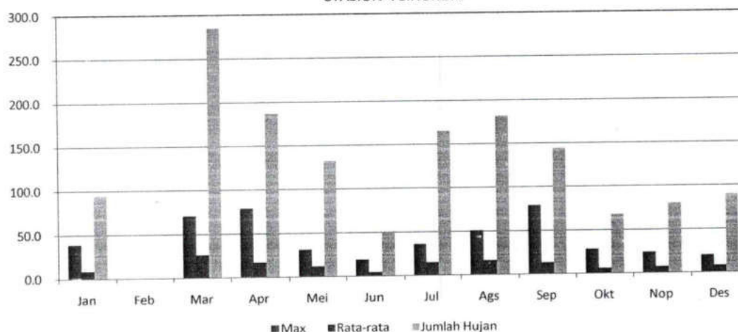
GRAFIK : CURAH HUJAN PRIODE 10 HARIAN 3 (MM) STASIUN : SINURUIK
