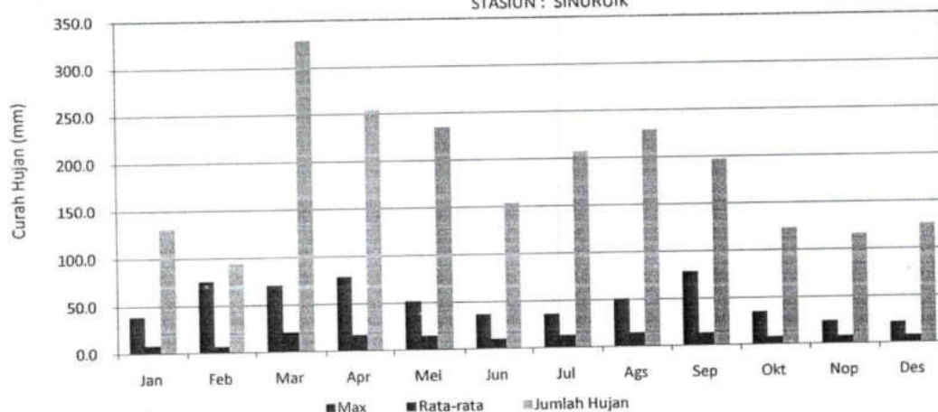
GRAFIK : CURAH HUJAN PRIODE (15 HARIAN 2) 2020 STASIUN : SINURUIK
