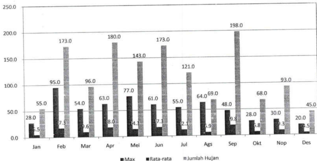
GRAFIK : CURAH HUJAN PRIODE 10 HARIAN 1 (MM) STASIUN : SINURUIK
