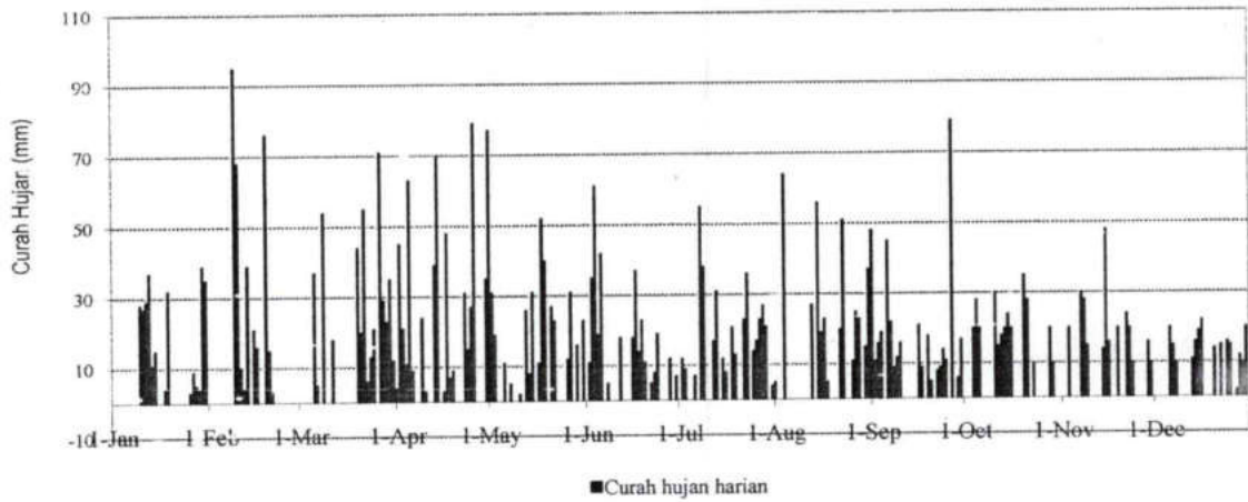
STATISTIK CURAH HUJAN HARIAN (MM) 2020 STASIUN : SINURUIK
