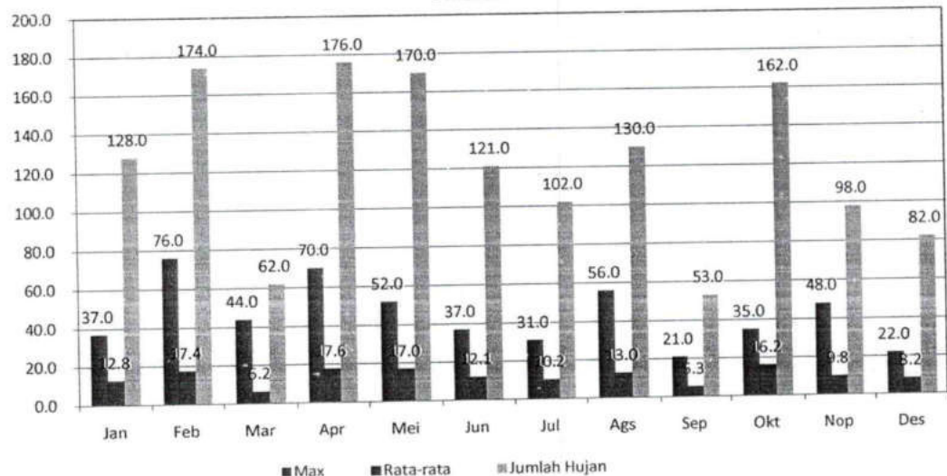
GRAFIK : CURAH HUJAN PRIODE 10 HARIAN 2 (MM) STASIUN : SINURUIK
