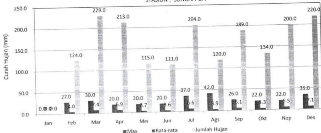
GRAFIK : CURAH HUJAN PRIODE BULANAN (MM) 2020 STASIUN : SUNGAI PUA
