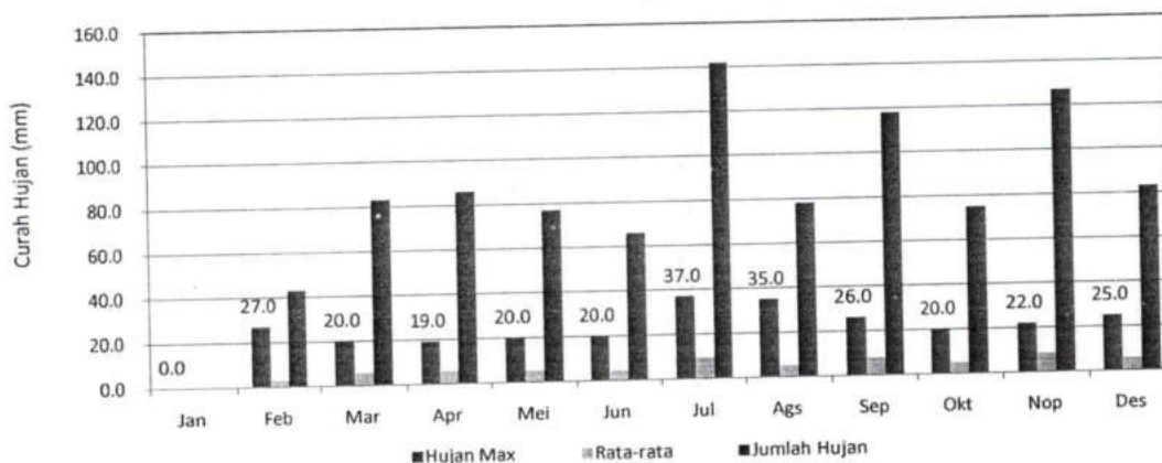
GRAFIK : CURAH HUJAN PRIODE ( 15 HARIAN 1) 2020 STASIUN : SUNGAI PUA
