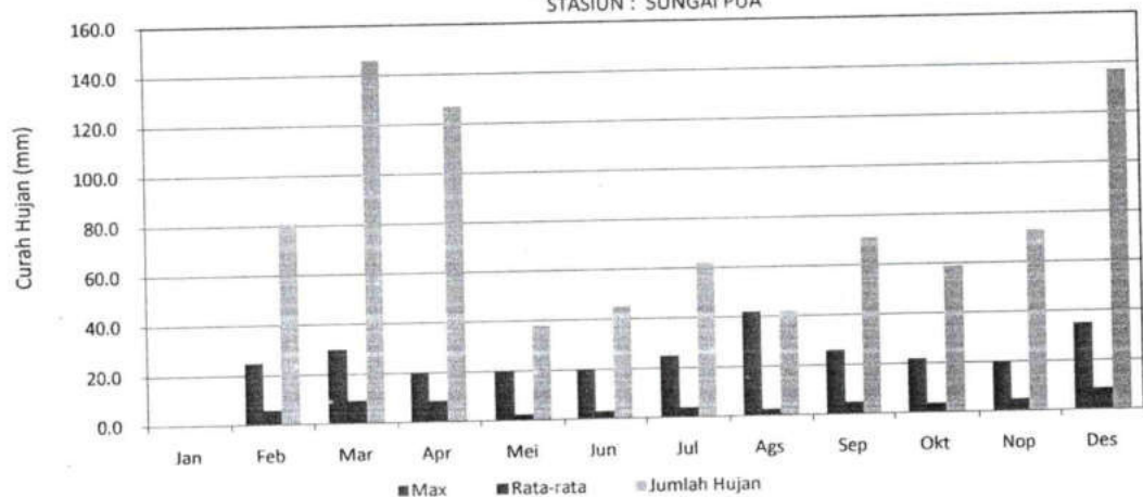
GRAFIK : CURAH HUJAN PRIODE (15 HARIAN 2) 2020 STASIUN : SUNGAI PUA
