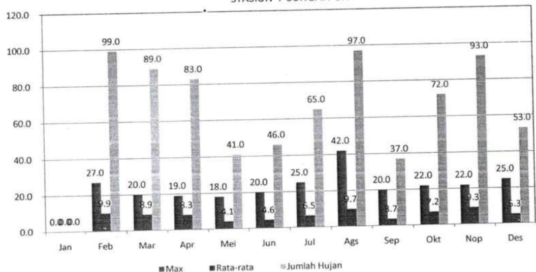
GRAFIK : CURAH HUJAN PRIODE 10 HARIAN 2 (MM) STASIUN : SUNGAI PUA
