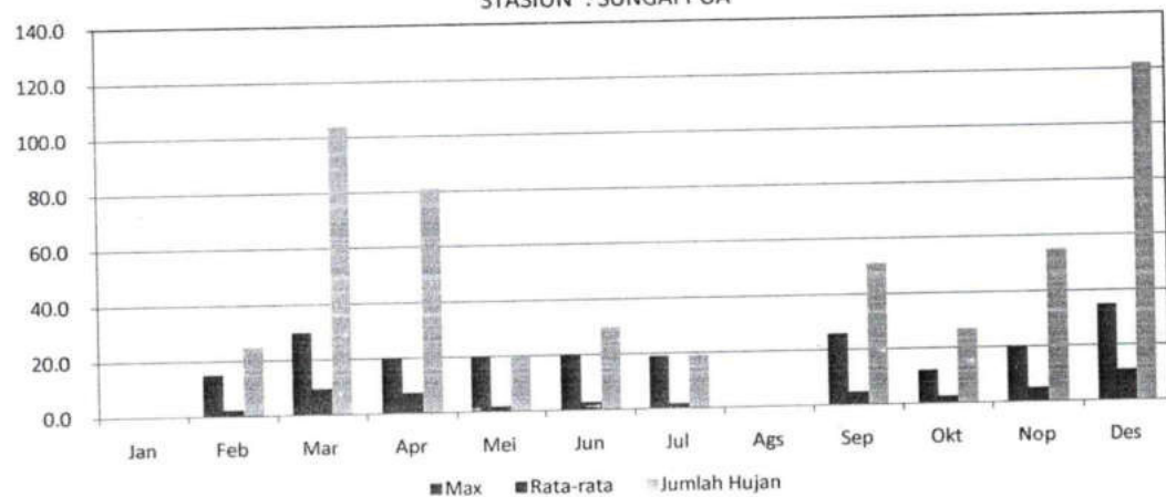
GRAFIK : CURAH HUJAN PRIODE 10 HARIAN 3 (MM) STASIUN : SUNGAI PUA
