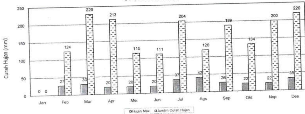
GRAFIK : HUJAN MAX DAN JUMLAH HUJAN BULANAN (MM) 2020 STASIUN : SUNGAI PUA
