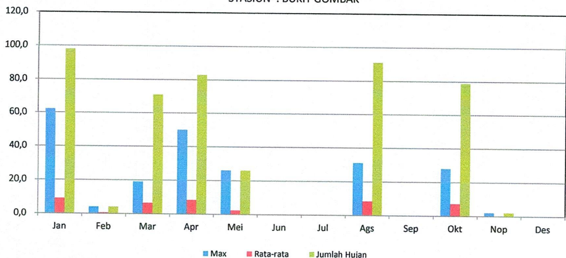
GRAFIK : CURAH HUJAN PRIODE 10 HARIAN 3 (MM) STASIUN : BUKIT GOMBAK
