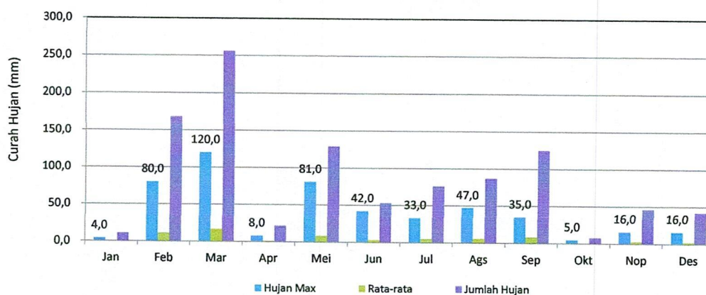
GRAFIK : CURAH HUJAN PRIODE ( 15 HARIAN 1) 2021 STASIUN : BUKIT GOMBAK
