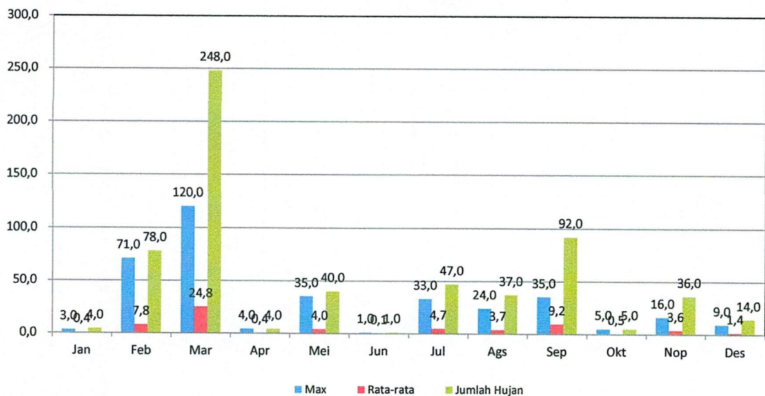
GRAFIK : CURAH HUJAN PRIODE 10 HARIAN 1 (MM) STASIUN : BUKIT GOMBAK
