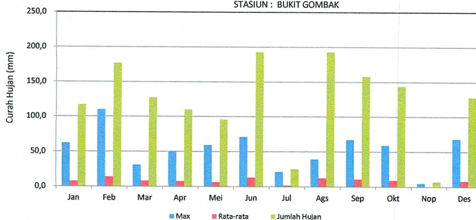
GRAFIK : CURAH HUJAN PRIODE (15 HARIAN 2) 2021 STASIUN : BUKIT GOMBAK
