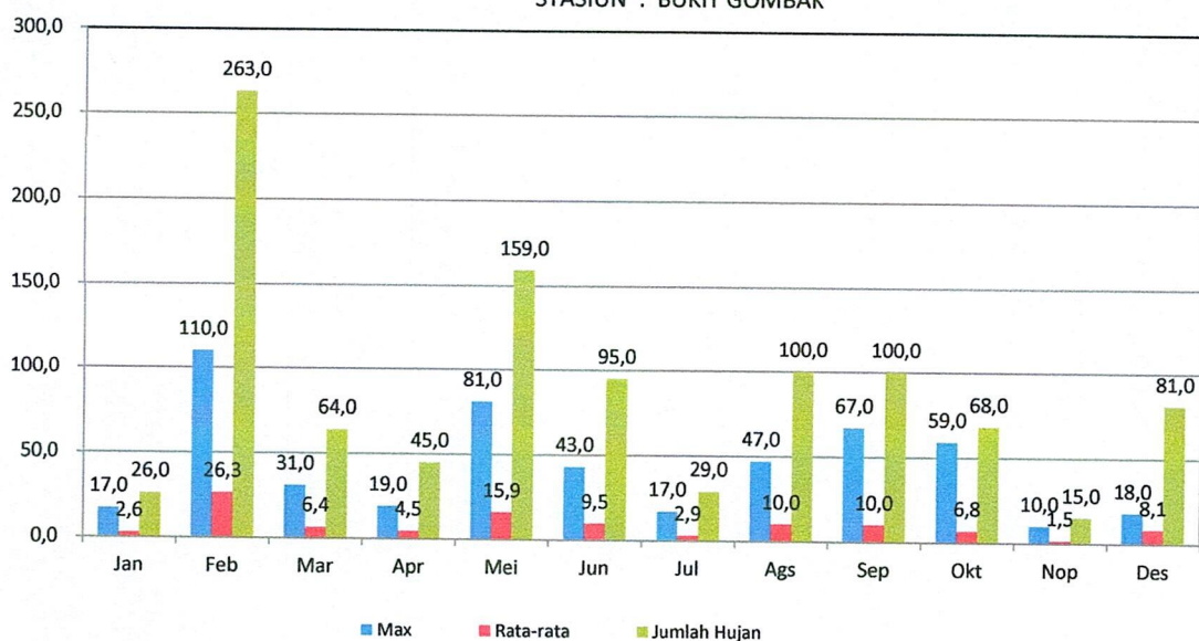
GRAFIK : CURAH HUJAN PRIODE 10 HARIAN 2 (MM) STASIUN : BUKIT GOMBAK
