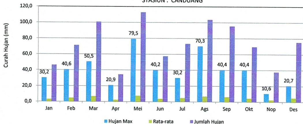
GRAFIK : CURAH HUJAN PRIODE ( 15 HARIAN 1) 2021 STASIUN : CANDUANG
