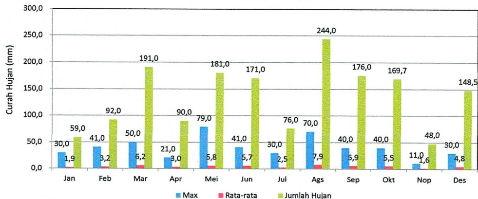
GRAFIK : CURAH HUJAN PRIODE BULANAN (MM) 2021 STASIUN : CANDUANG
