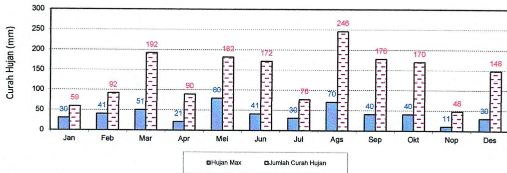
GRAFIK : HUJAN MAX DAN JUMLAH HUJAN BULANAN (MM) 2021 STASIUN : CANDUANG
