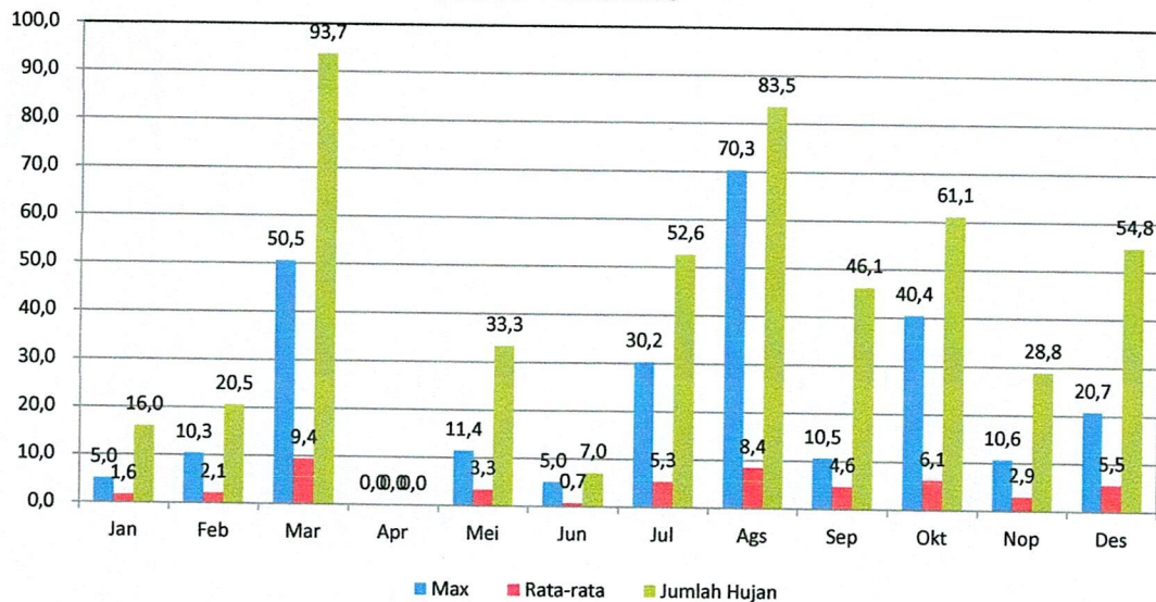
GRAFIK : CURAH HUJAN PRIODE 10 HARIAN 1 (MM) STASIUN : CANDUANG
