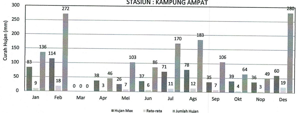
GRAFIK : CURAH HUJAN PRIODE ( 15 HARIAN 1) 2021 STASIUN : KAMPUNG AMPAT
