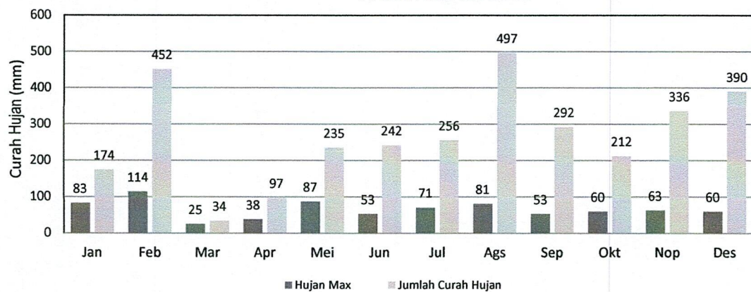
GRAFIK : HUJAN MAX DAN JUMLAH HUJAN BULANAN (MM) 2021 STASIUN : KAMPUNG AMPAT
