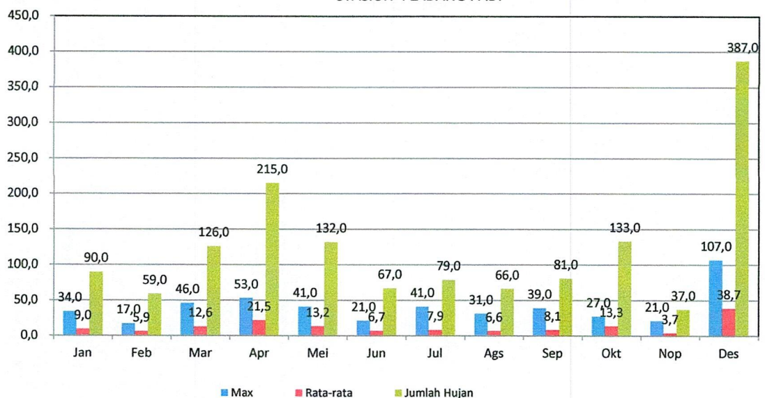
GRAFIK : CURAH HUJAN PRIODE 10 HARIAN 2 (MM) STASIUN : LADANG PADI
