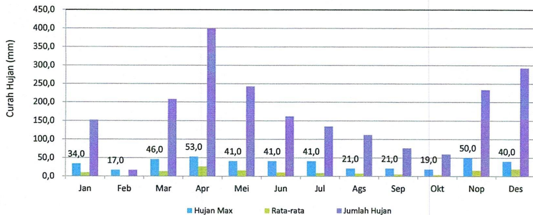
GRAFIK : CURAH HUJAN PRIODE ( 15 HARIAN 1) 2021 STASIUN : LADANG PADI
