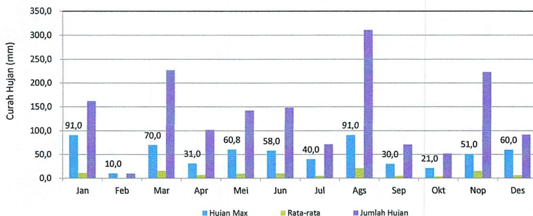
GRAFIK : CURAH HUJAN PRIODE ( 15 HARIAN 1) 2021 STASIUN : LIMAU MANIS
