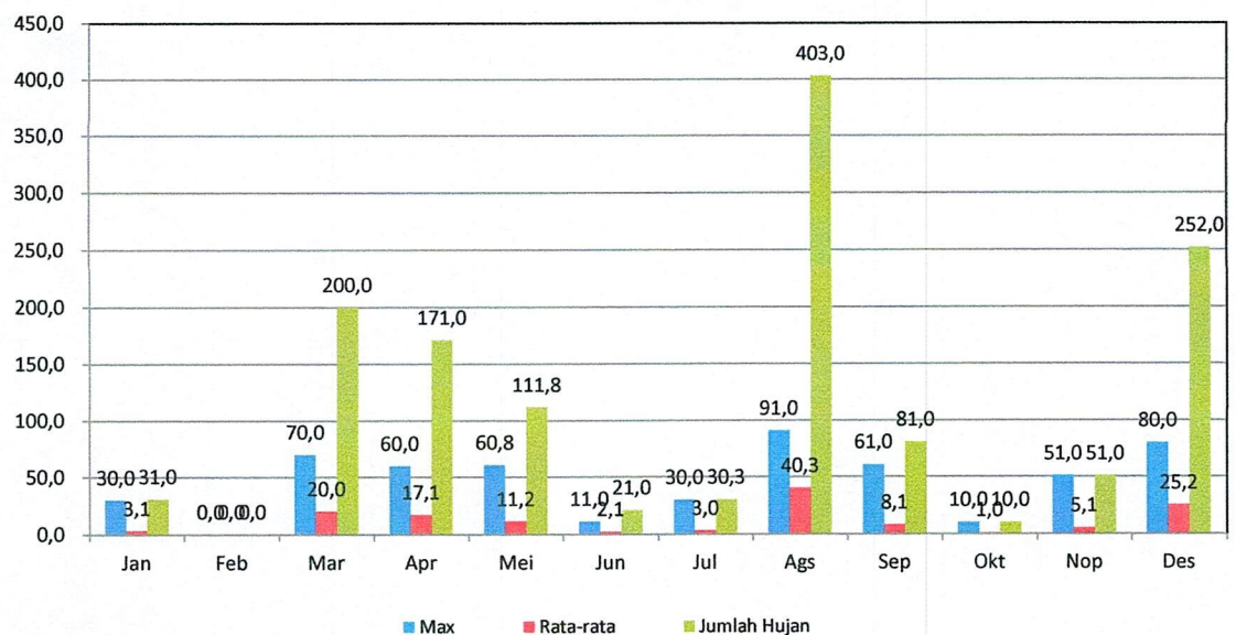
GRAFIK : CURAH HUJAN PRIODE 10 HARIAN 2 (MM) STASIUN : Limau Manis
