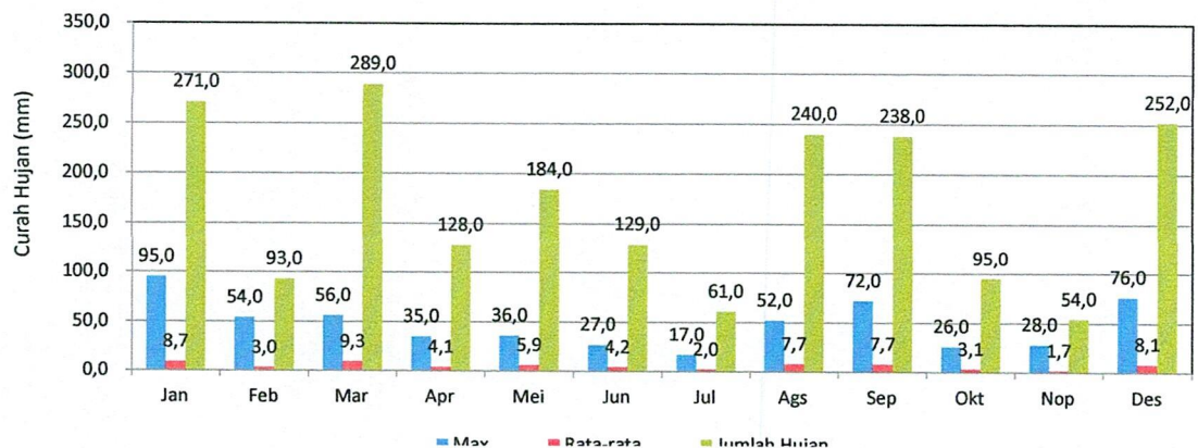
GRAFIK : CURAH HUJAN PRIODE BULANAN (MM) 2021 STASIUN : RAO
