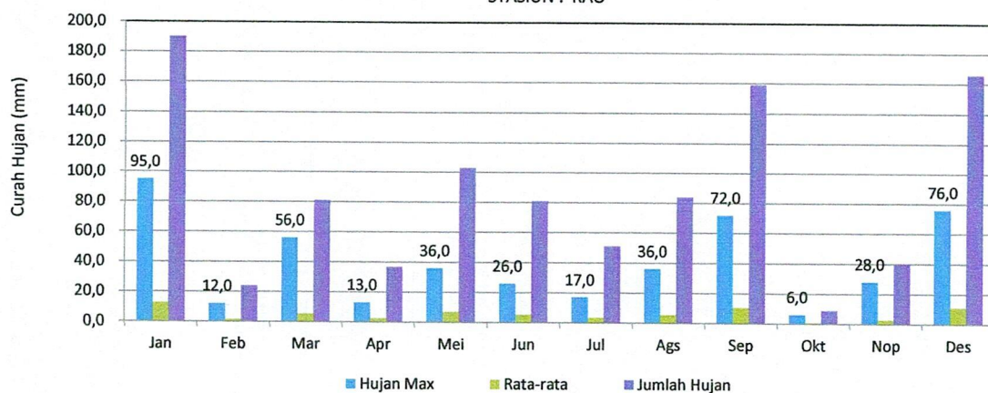
GRAFIK : CURAH HUJAN PRIODE ( 15 HARIAN 1) 2021 STASIUN : RAO
