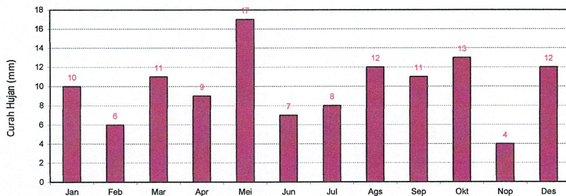
GRAFIK : JUMLAH HARI HUJAN (MM) 2021 STASIUN : RAO
