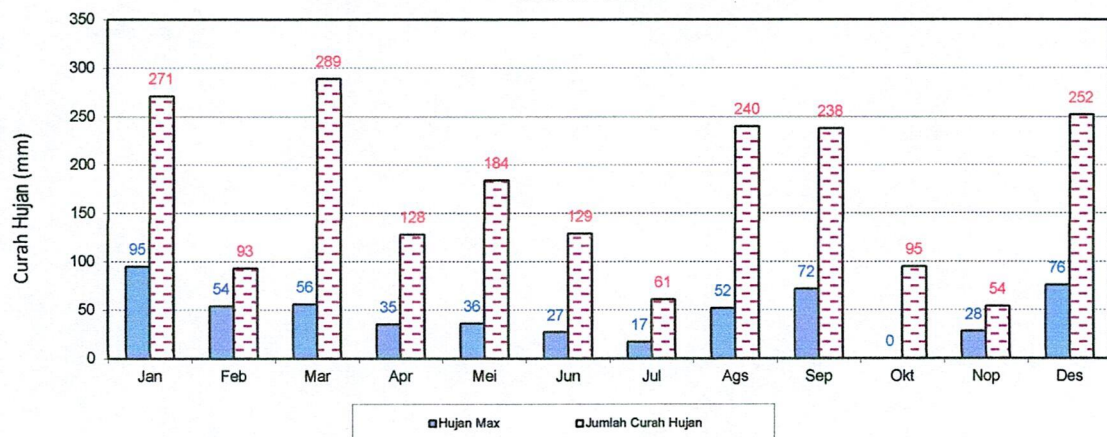
GRAFIK : HUJAN MAX DAN JUMLAH HUJAN BULANAN (MM) 2021 STASIUN : RAO
