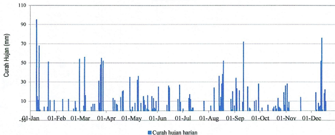
STATISTIK CURAH HUJAN HARIAN (MM) 2021 STASIUN : RAO
