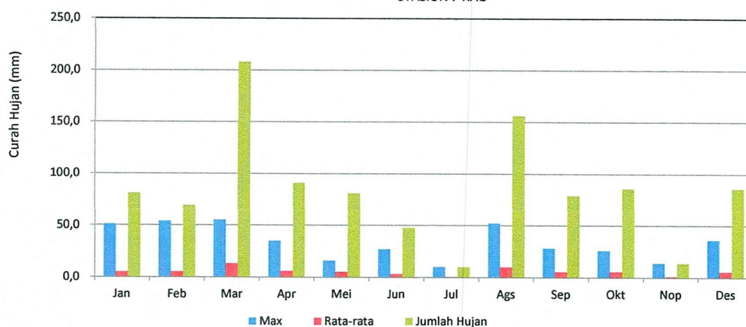
GRAFIK : CURAH HUJAN PRIODE (15 HARIAN 2) 2021 STASIUN : RAO
