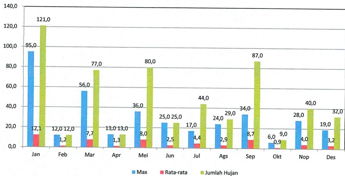
GRAFIK : CURAH HUJAN PRIODE 10 HARIAN 1 (MM) STASIUN : RAO
