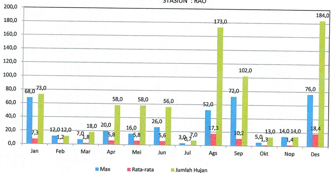
GRAFIK : CURAH HUJAN PRIODE 10 HARIAN 2 (MM) 2021 STASIUN : RAO
