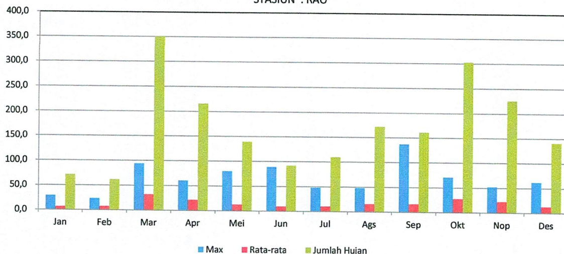
GRAFIK : CURAH HUJAN PRIODE 10 HARIAN 3 (MM)
