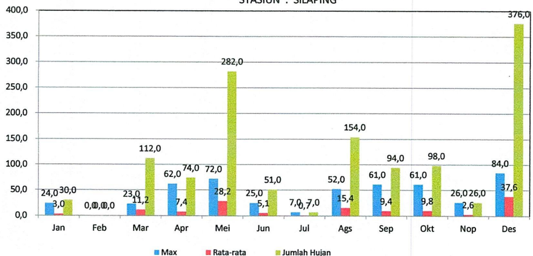
GRAFIK : CURAH HUJAN PRIODE 10 HARIAN 2 (MM) 2021 STASIUN : SILAPING
