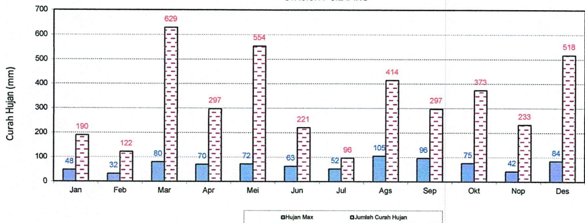
GRAFIK : HUJAN MAX DAN JUMLAH HUJAN BULANAN (MM) 2021 STASIUN : SILAPING
