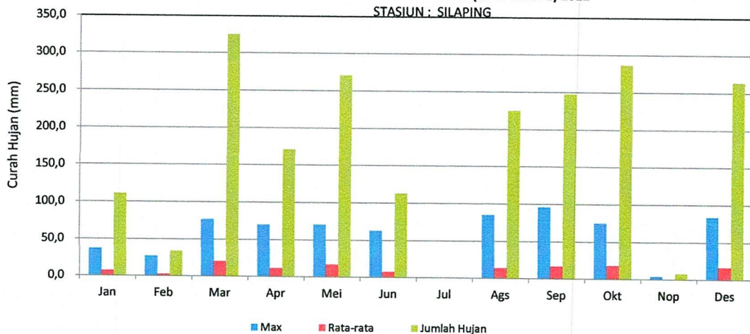
GRAFIK : CURAH HUJAN PRIODE (15 HARIAN 2) 2021 STASIUN : SILAPING
