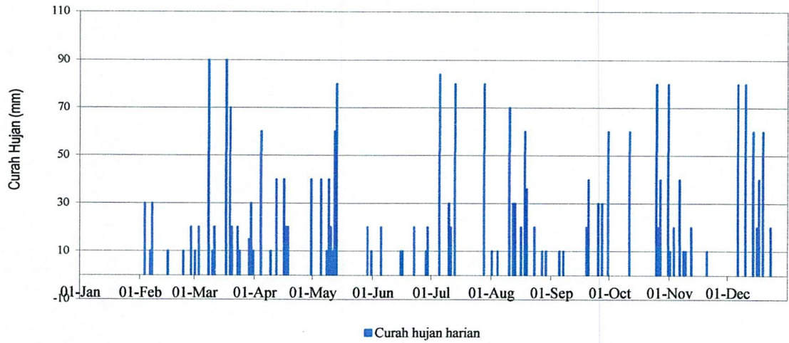
STATISTIK CURAH HUJAN HARIAN (MM) 2021 STASIUN : SUKA MENANTI- BENDUNG TONGAR
