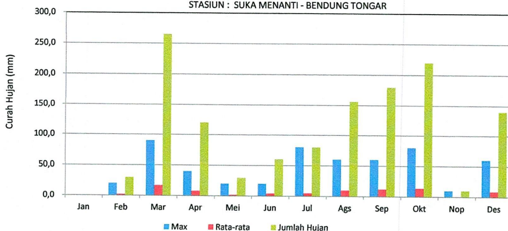
GRAFIK : CURAH HUJAN PRIODE (15 HARIAN 2) 2021 STASIUN : SUKA MENANTI - BENDUNG TONGAR
