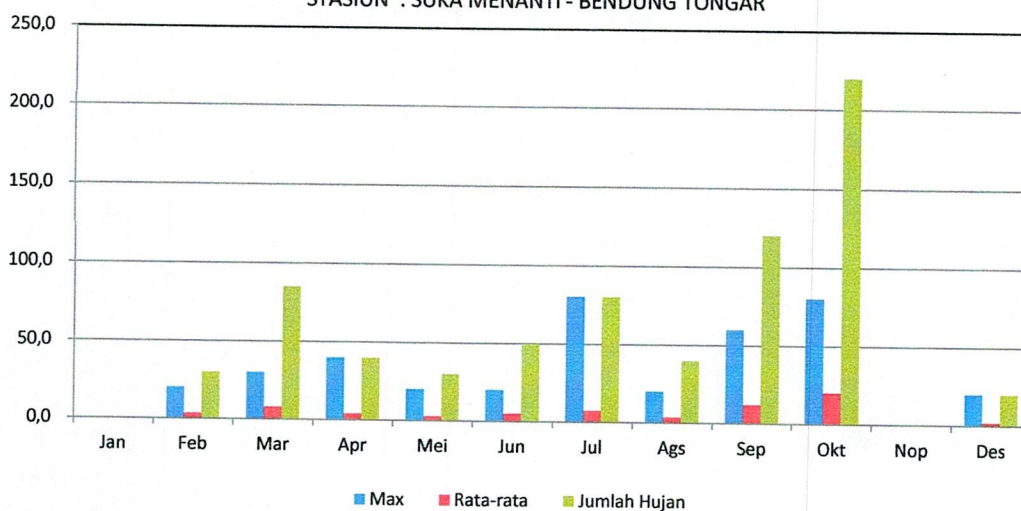
GRAFIK : CURAH HUJAN PRIODE 10 HARIAN 3 (MM) STASIUN : SUKA MENANTI - BENDUNG TONGAR
