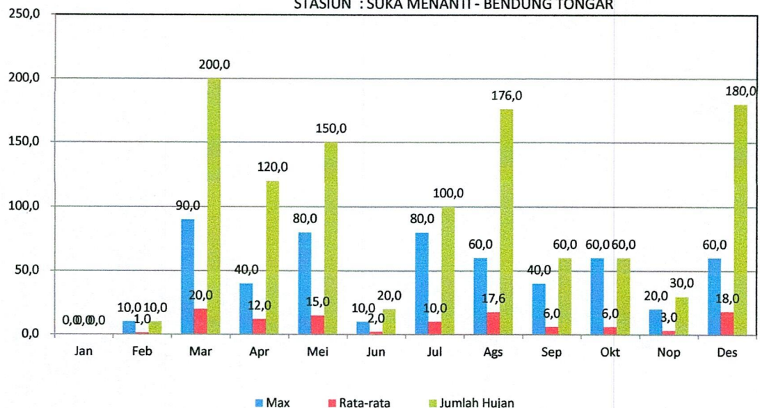
GRAFIK : CURAH HUJAN PRIODE 10 HARIAN 2 (MM) STASIUN : SUKA MENANTI - BENDUNG TONGAR
