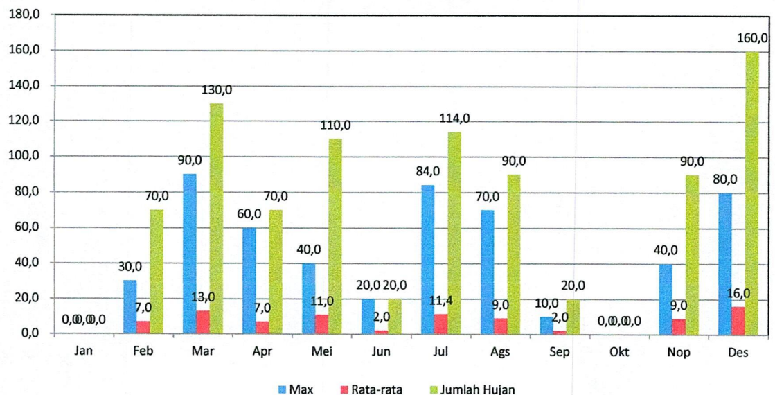
GRAFIK : CURAH HUJAN PRIODE 10 HARIAN 1 (MM) STASIUN : SUKA MENANTI - BENDUNG TONGAR
