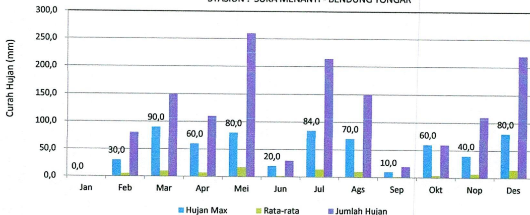
GRAFIK : CURAH HUJAN PRIODE ( 15 HARIAN 1) 2021 STASIUN : SUKA MENANTI - BENDUNG TONGAR
