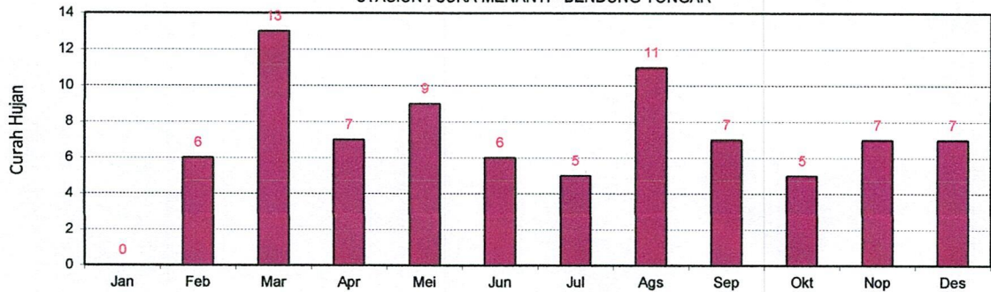
GRAFIK : JUMLAH HARI HUJAN (MM) 2021 STASIUN : SUKA MENANTI- BENDUNG TONGAR
