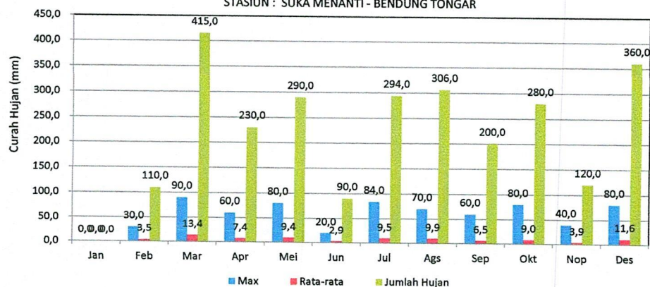
GRAFIK : CURAH HUJAN PRIODE BULANAN (MM) 2021
