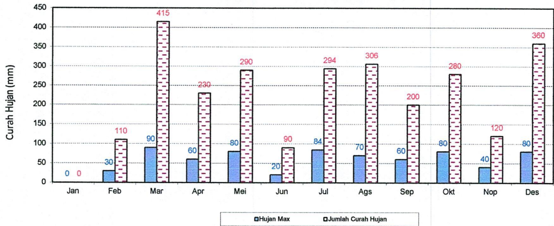
GRAFIK : JUMLAH HARI HUJAN (MM) 2021 STASIUN : SUKA MENANTI- BENDUNG TONGAR
