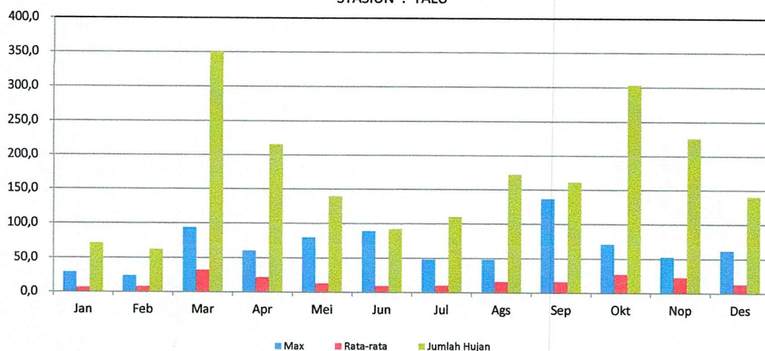
GRAFIK : CURAH HUJAN PRIODE 10 HARIAN 3 (MM) 2021 STASIUN : TALU
