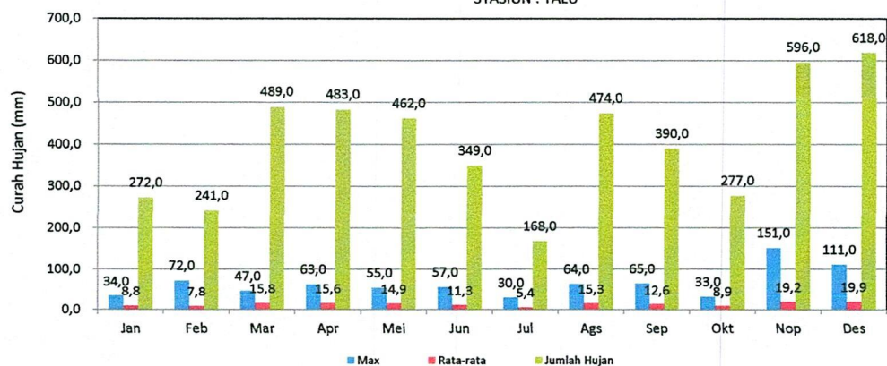
GRAFIK : CURAH HUJAN PRIODE BULANAN (MM) 2021
