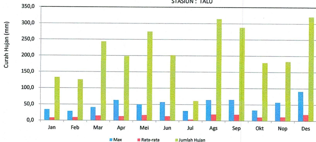
GRAFIK : CURAH HUJAN PRIODE (15 HARIAN 2) 2021 STASIUN : TALU
