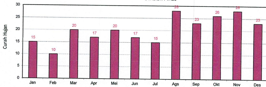
GRAFIK : JUMLAH HARI HUJAN (MM) 2021 STASIUN : TALU
