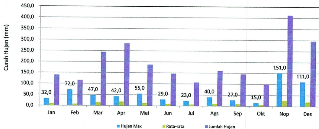
GRAFIK : CURAH HUJAN PRIODE ( 15 HARIAN 1) 2021 STASIUN : TALU
