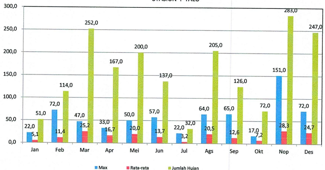
GRAFIK : CURAH HUJAN PRIODE 10 HARIAN 2 (MM) 2021 STASIUN : TALU
