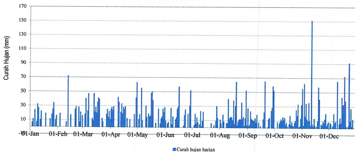
STATISTIK CURAH HUJAN HARIAN (MM) 2021 STASIUN : TALU
