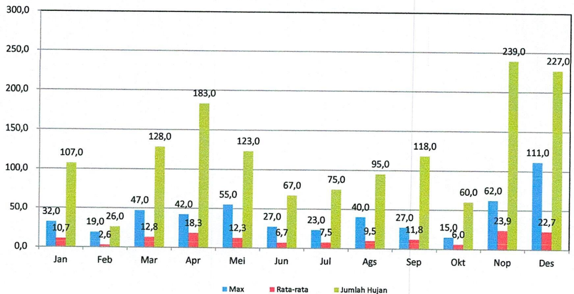
GRAFIK : CURAH HUJAN PRIODE 10 HARIAN 1 (MM) 2021 STASIUN : TALU
