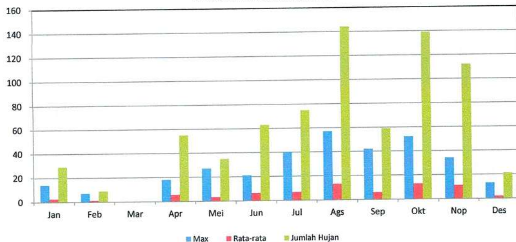
GRAFIK : CURAH HUJAN PRIODE 10 HARIAN 3 (MM) 2022 STASIUN : BALINGKA SIANOK.
