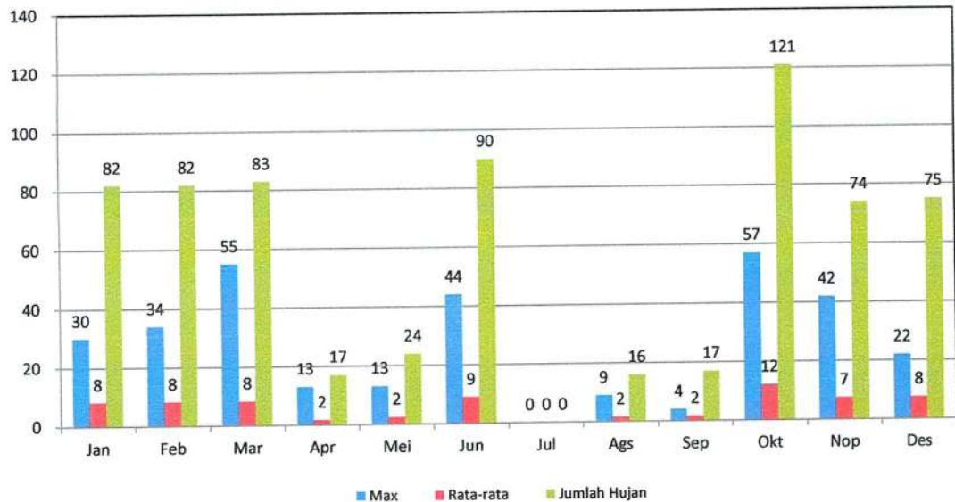
GRAFIK : CURAH HUJAN PRIODE 10 HARIAN 1 (MM) 2022 STASIUN : BALINGKA SIANOK.
