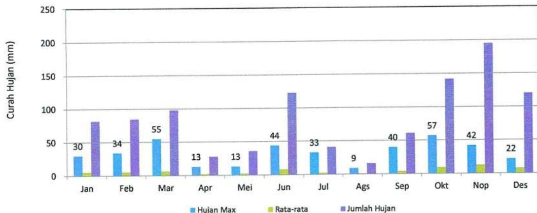
GRAFIK : CURAH HUJAN PRIODE ( 15 HARIAN 1) 2022 STASIUN : BALINGKA SIANOK
