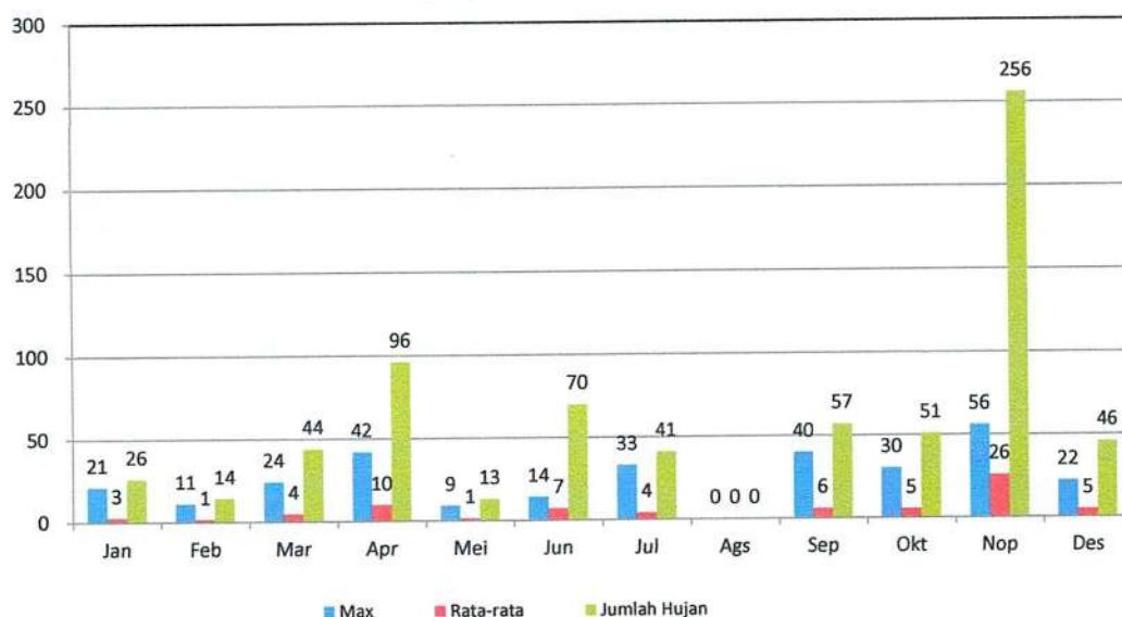
GRAFIK : CURAH HUJAN PRIODE 10 HARIAN 2 (MM) 2022 STASIUN : BALINGKA SIANOK.
