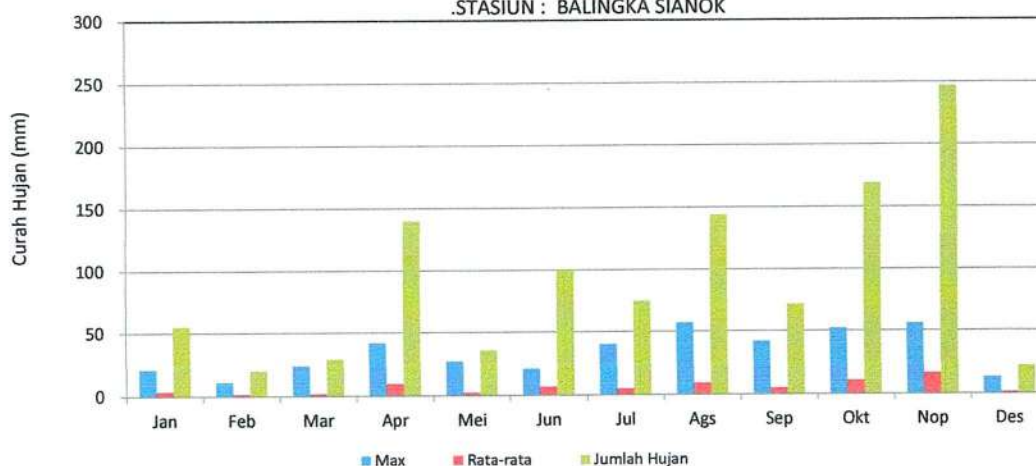
GRAFIK : CURAH HUJAN PRIODE (15 HARIAN 2) 2022 STASIUN : BALINGKA SIANOK
