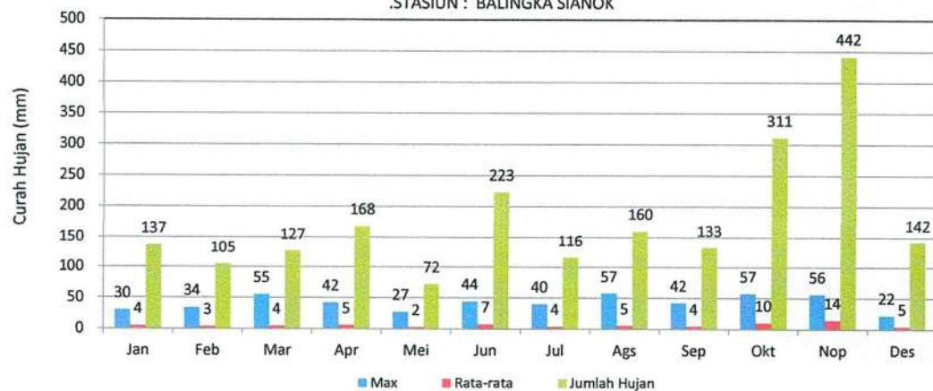
GRAFIK : CURAH HUJAN PRIODE BULANAN (MM) 2022
