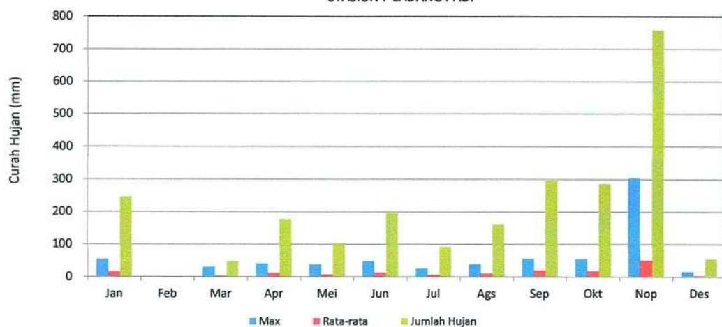
GRAFIK : CURAH HUJAN PRIODE (15 HARIAN 2) 2022 STASIUN : LADANG PADI
