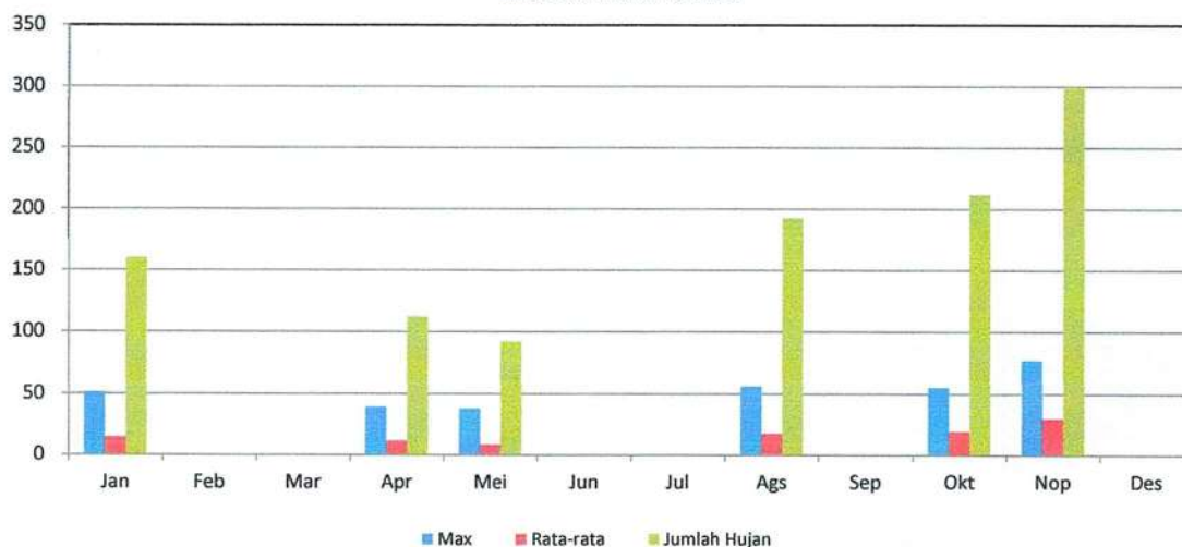
GRAFIK : CURAH HUJAN PRIODE 10 HARIAN 3 (MM) 2022 STASIUN : LADANG PADI
