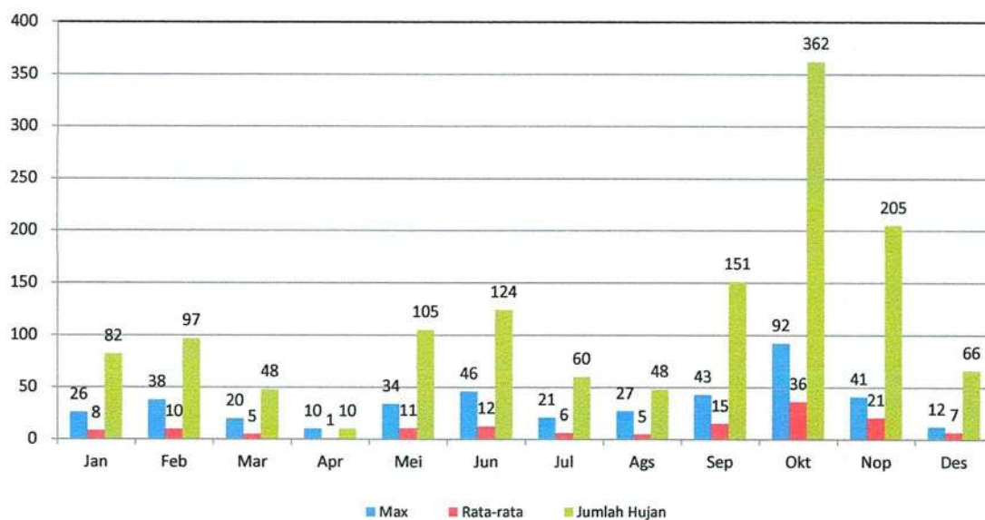
GRAFIK : CURAH HUJAN PRIODE 10 HARIAN 1 (MM) 2022 STASIUN : LADANG PADI
