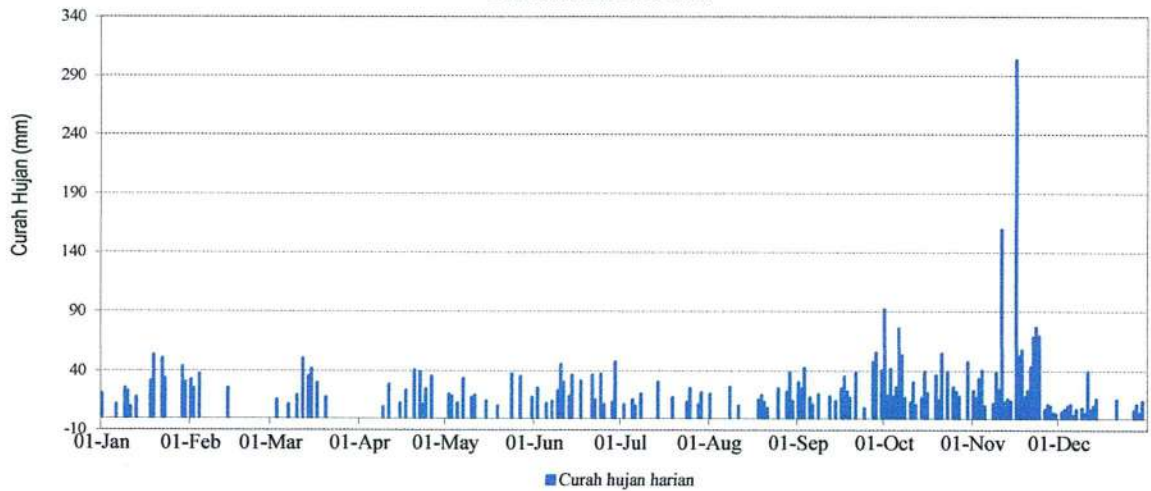
STATISTIK CURAH HUJAN HARIAN (MM) 2022 STASIUN : LADANG PADI
