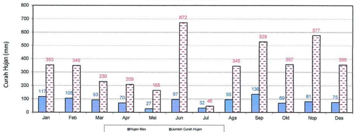
GRAFIK : HUJAN MAX DAN JUMLAH HUJAN BULANAN (MM) 2022 STASIUN : PARAMAN TALANG
