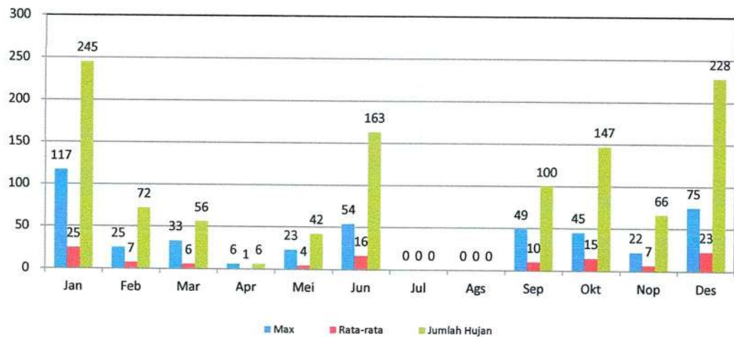
GRAFIK : CURAH HUJAN PRIODE 10 HARIAN 1 (MM) STASIUN : PARAMAN TALANG
