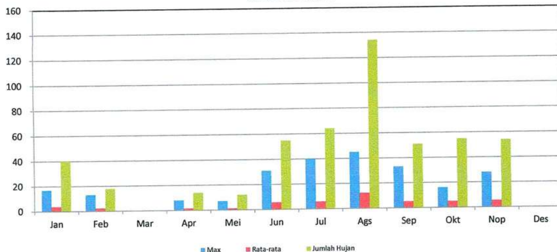
GRAFIK : CURAH HUJAN PRIODE 10 HARIAN 3 (MM) 2022 STASIUN : SULIKI
