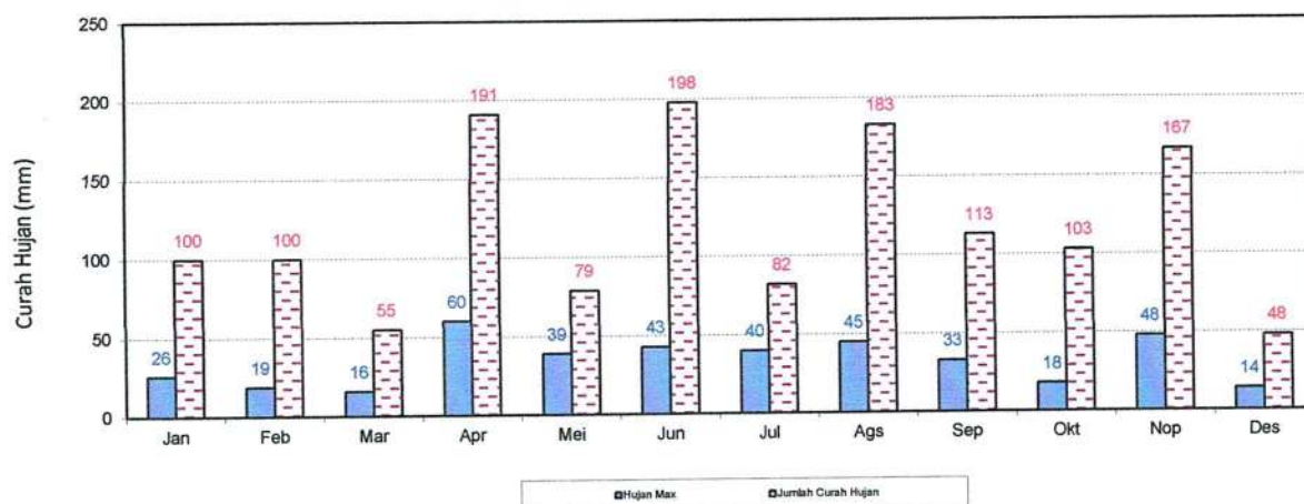
GRAFIK : HUJAN MAX DAN JUMLAH HUJAN BULANAN (MM) 2022
