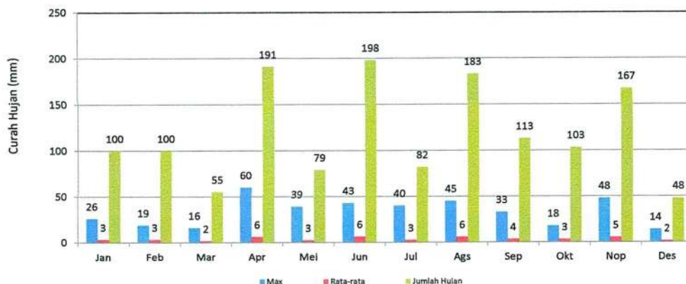
GRAFIK : CURAH HUJAN PRIODE BULANAN (MM) 2022 STASIUN : SULIKI
