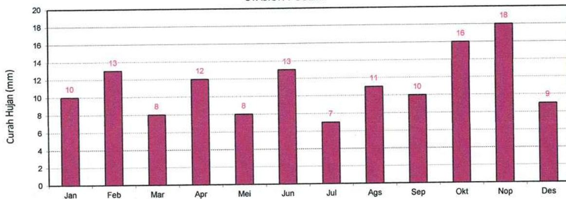
GRAFIK : JUMLAH HARI HUJAN (MM) 2022 STASIUN : SULIKI
