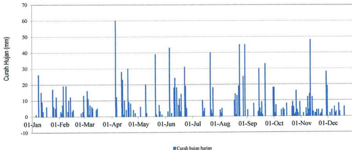
STATISTIK CURAH HUJAN HARIAN (MM) 2022 STASIUN : SULIKI
