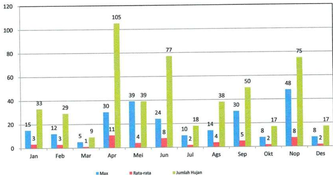
GRAFIK : CURAH HUJAN PRIODE 10 HARIAN 2 (MM) 2022 STASIUN : SULIKI
