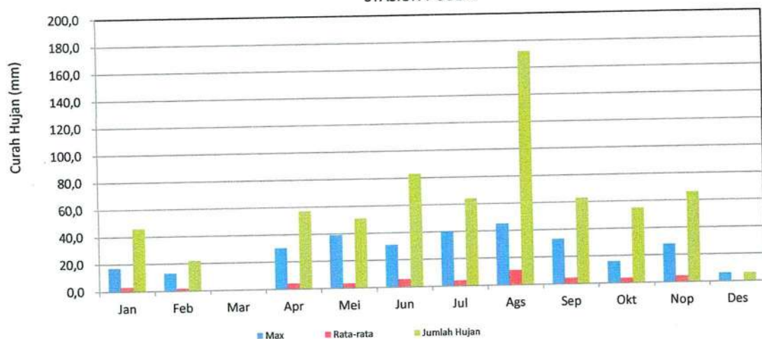
GRAFIK : CURAH HUJAN PRIODE (15 HARIAN 2) 2022 STASIUN : SULIKI
