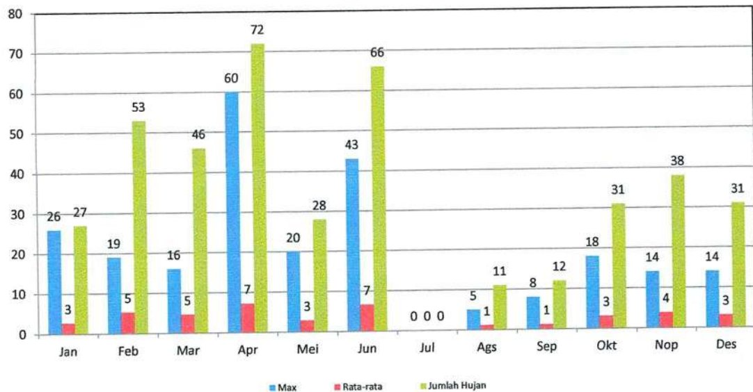
GRAFIK : CURAH HUJAN PRIODE 10 HARIAN 1 (MM) 2022 STASIUN : SULIKI
