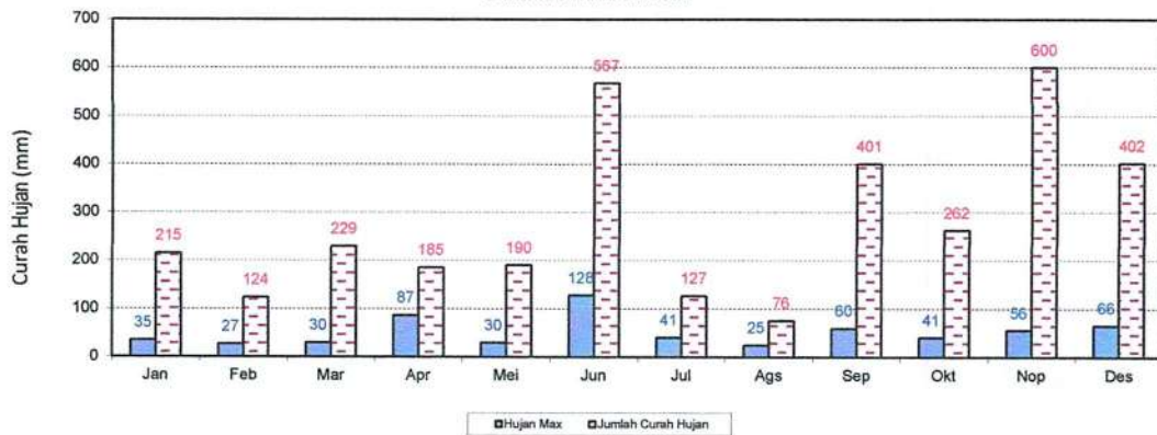
GRAFIK : HUJAN MAX DAN JUMLAH HUJAN BULANAN (MM) 2022 STASIUN : SUNGAI PUA
