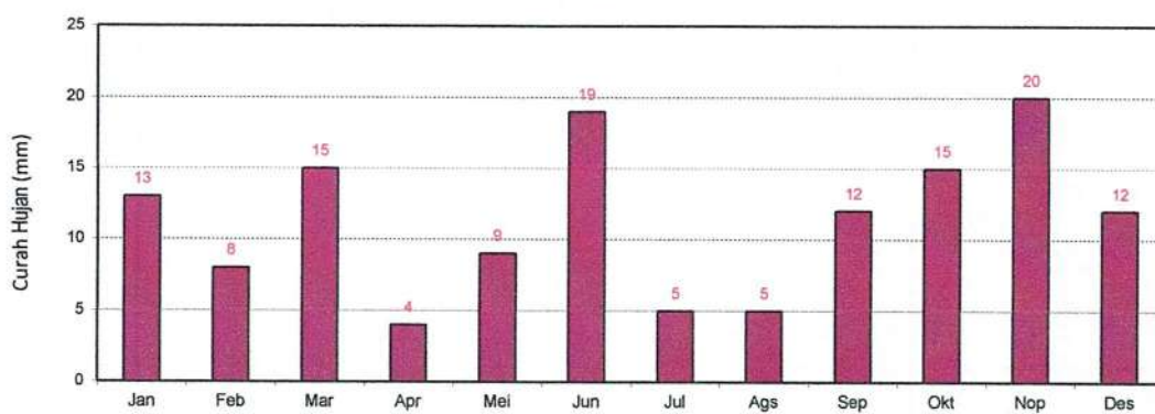
GRAFIK : JUMLAH HARI HUJAN (MM) 2022 STASIUN : SUNGAI PUA
