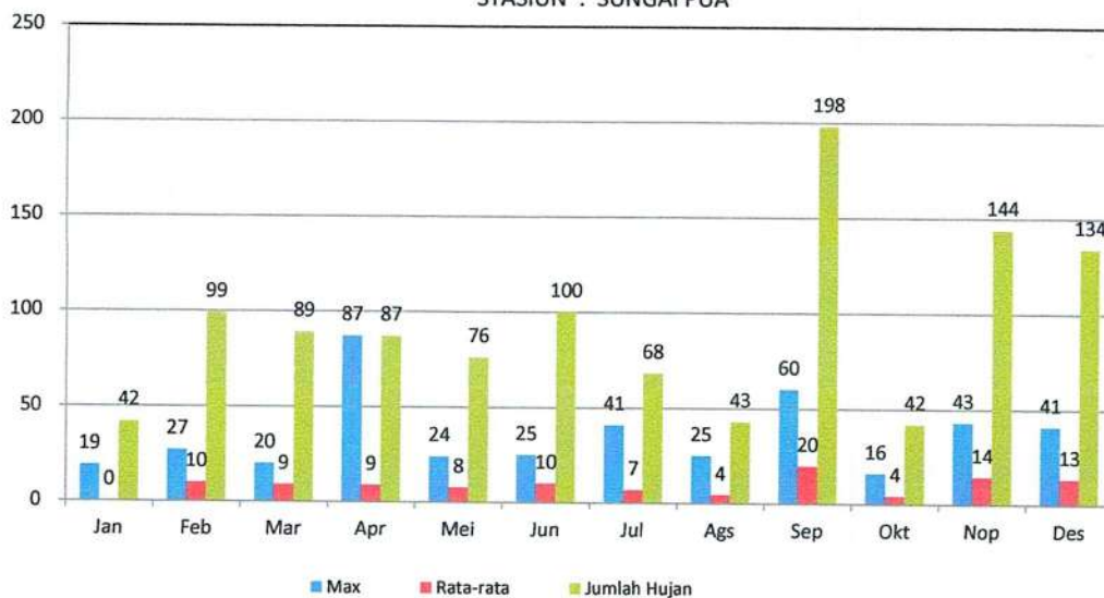
GRAFIK : CURAH HUJAN PRIODE 10 HARIAN 2 (MM) STASIUN : SUNGAI PUA
