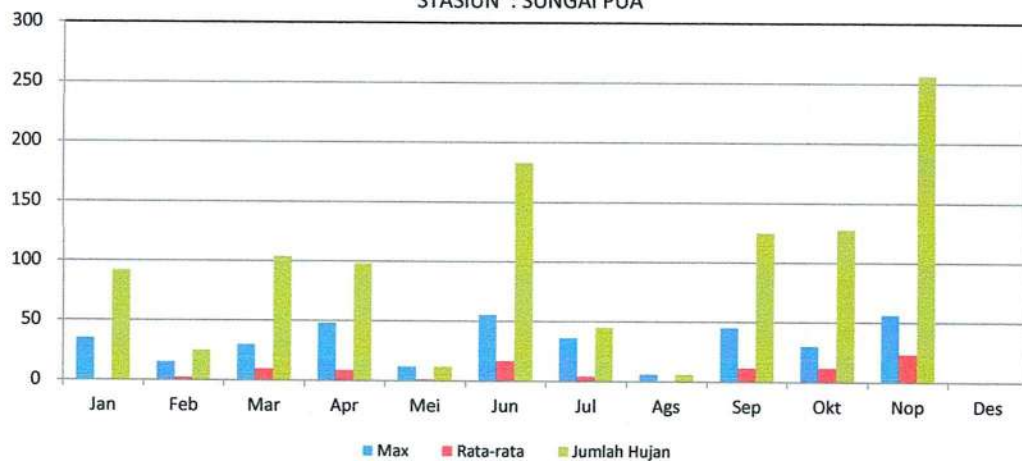
GRAFIK : CURAH HUJAN PRIODE 10 HARIAN 3 (MM) STASIUN : SUNGAI PUA
