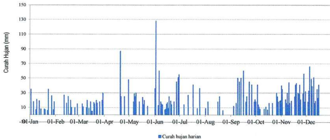
STATISTIK CURAH HUJAN HARIAN (MM) 2022 STASIUN : SUNGAI PUA
