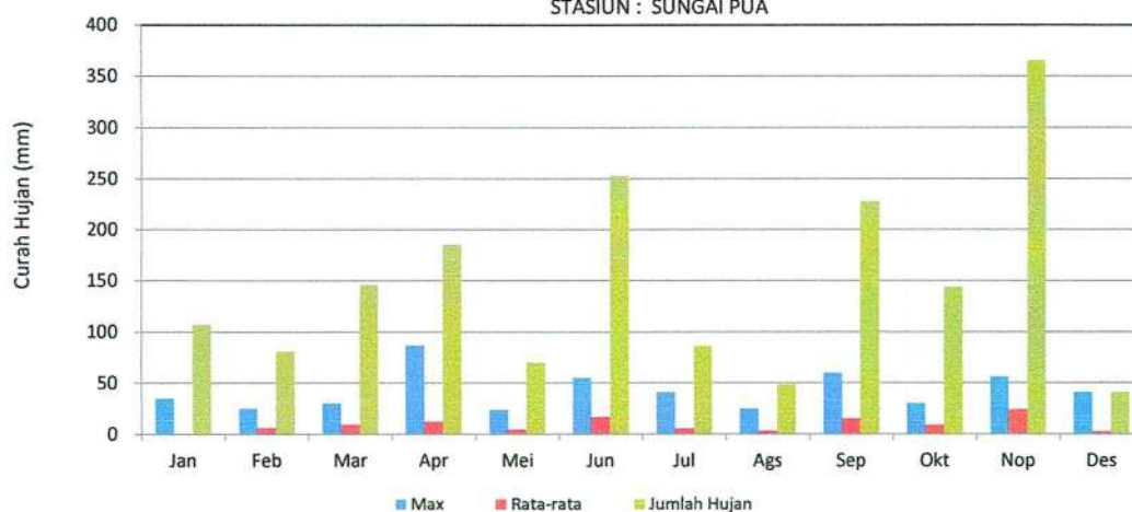
GRAFIK : CURAH HUJAN PRIODE (15 HARIAN 2) 2022 STASIUN : SUNGAI PUA
