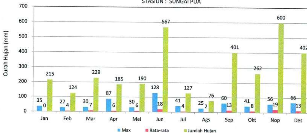
GRAFIK : CURAH HUJAN PRIODE BULANAN (MM) 2022
