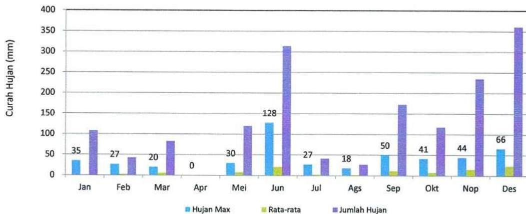
GRAFIK : CURAH HUJAN PRIODE ( 15 HARIAN 1) 2022 STASIUN : SUNGAI PUA
