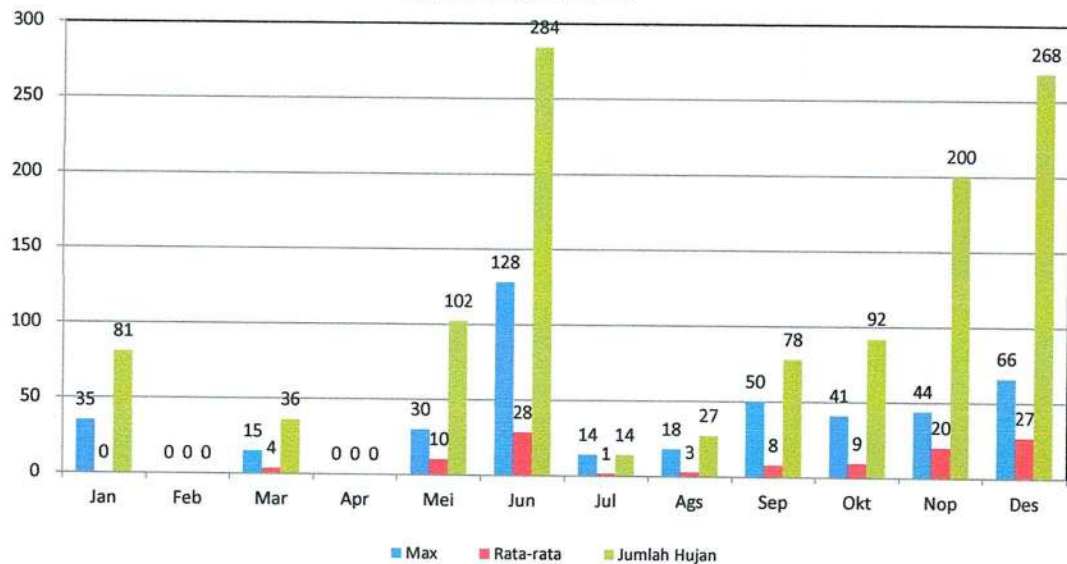
GRAFIK : CURAH HUJAN PRIODE 10 HARIAN 1 (MM) STASIUN : SUNGAI PUA
